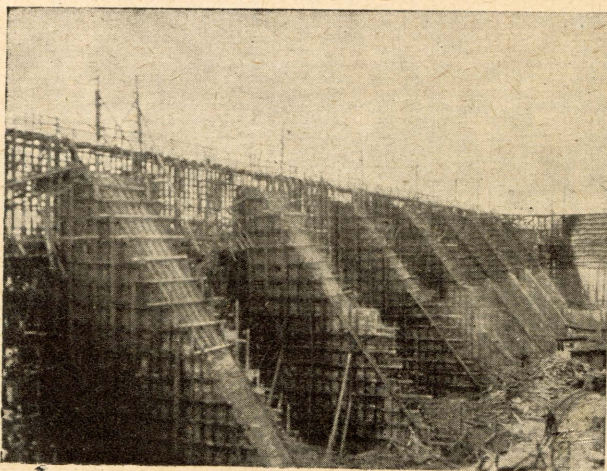
Część budowanej na Dźwinie zapory wodnej w Kegums
