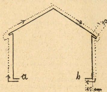
Rys. 5. Sposób szycia ścian bocznych i dachu w przekroju
