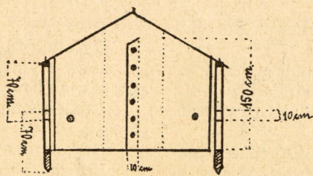
Rys. 2. Ściana przednia — zapięta
