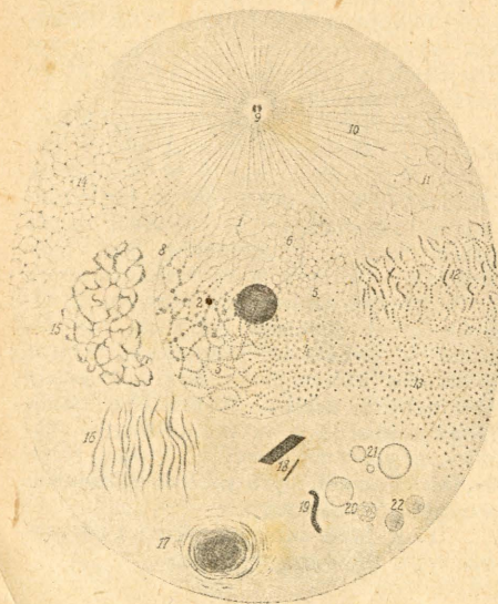
Schemat komórki (wielokrotne powiększenie)
