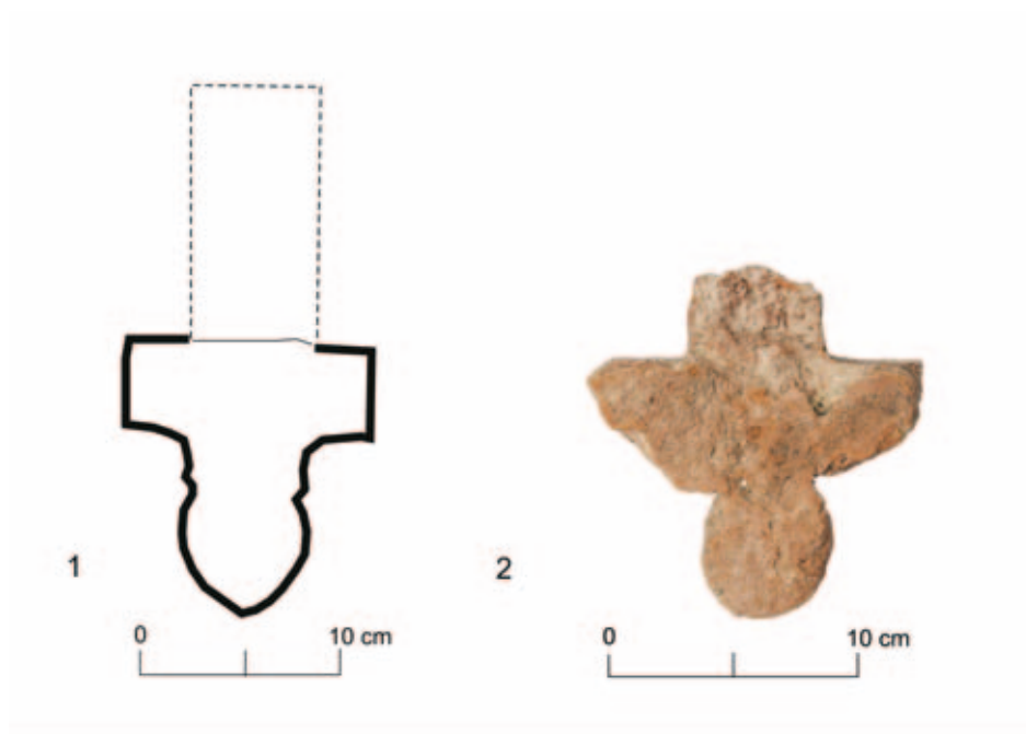
il. 12. Cegły profilowane żebrowo-sklepieniowe. 1. Przykład destrukcji żebra z wpustem; katedra w Kołobrzegu, sklepienie pod emporami nawy północnej, pomiar J.T. Frazik, źródło: J.T. Frazik, dz. cyt., s. 35, ryc. 17. 2. Tykocin, st. 38, tzw. kępa bernardyńska. Fragment cegły profilowanej żebrowo-sklepieniowej (fot. A. Sierko-Szymańska)
