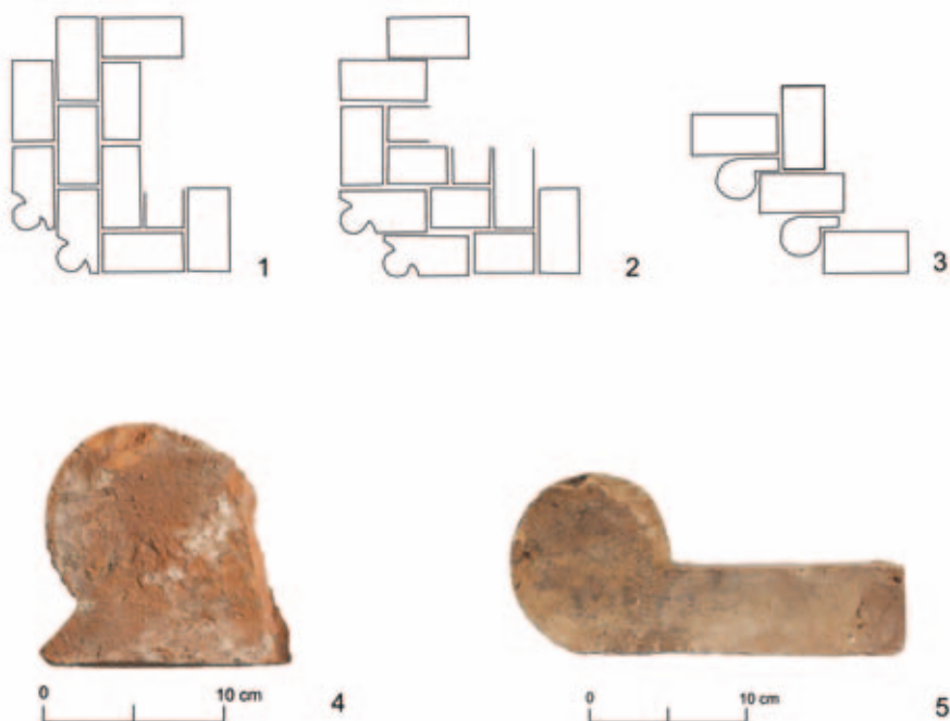
il. 11. Cegły profilowane ościeżnicowe. 1–2. Układ cegieł w ościeżu drzwi profilowanych w murze o grubości trzech cegieł (oprac. A. Kąsinowski), źródło: A. Kąsinowski, dz. cyt. s. 7, ryc. 15, B1, B2. 3. Profil okna kościoła w Kołbaczu z użyciem cegły specjalnej (oprac. A. Kąsinowski), źródło: A. Kąsinowski, dz. cyt., ryc. 15, C. 4. Tykocin, st. 38, tzw. kępa bernardyńska. Fragment cegły profilowanej ościeżnicowej (fot. A. Sierko-Szymańska). 5. Supraśl. Monaster oo. Bazylianów, cegła specjalna, ościeżnicowa (fot. A. Sierko-Szymańska)
