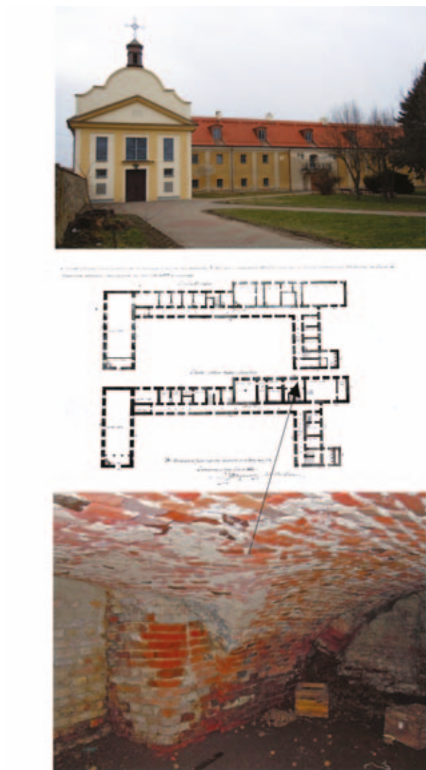
il. 5. Tykocin, gm. Tykocin, woj. podlaskie. Klasztor oo. Bernardynów, 1771–1793. 1. Widok na skrzydło wschodnie (kościół) i południowe od strony północnej. 2. Rysunek szkicowy parteru i I piętra założenia klasztornego z 1865 r. (AGAD Warszawa, sygn. 21-12.ark.2., neg. PKZ Warszawa nr 118077). 3. Piwnica w skrzydle południowym (fot. I. Taranta)
