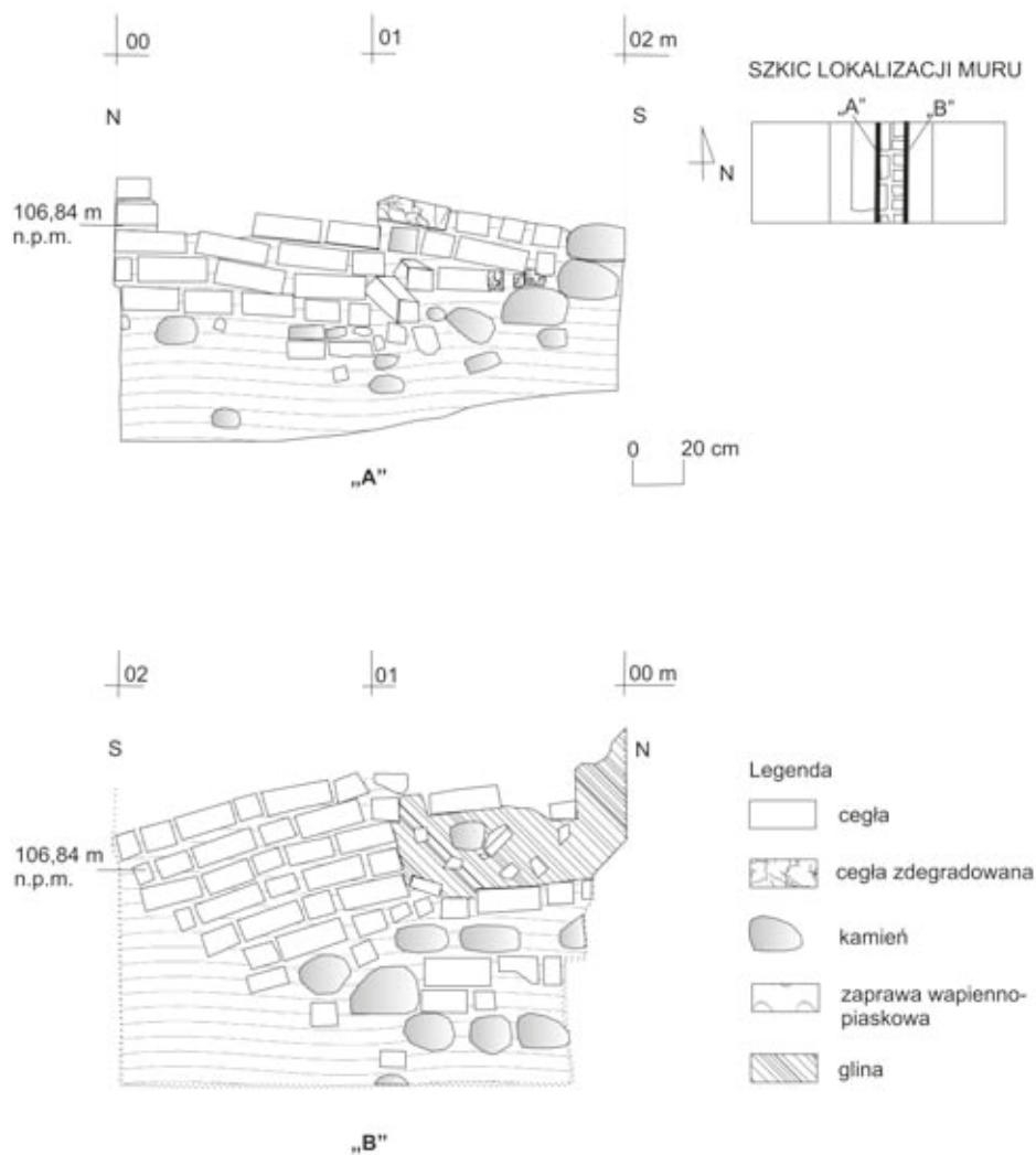
il. 6. Tykocin, st. 38, tzw. kępa bernardyńska, gm. Tykocin, woj. podlaskie. Wykop 1, odcinek C, mur ceglano-kamienny. „A” – lico W (rys. I. Taranta), „B” – lico E (rys. H. Karwowska, I. Taranta)
