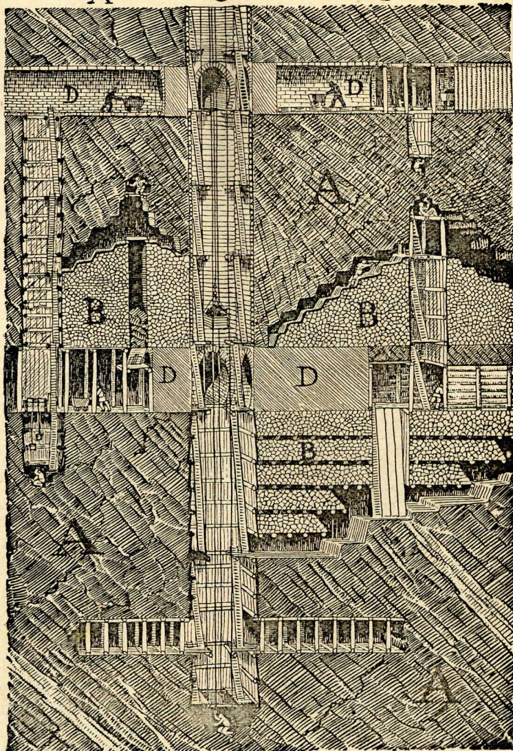
Wnętrze kopalni węgla. A — pokłady węgla. B — puste przestrzenie po wydobyciu węgla, zapełnione piaskiem albo gruzem. C — szyb pionowy. D — chodnik poziomy.
