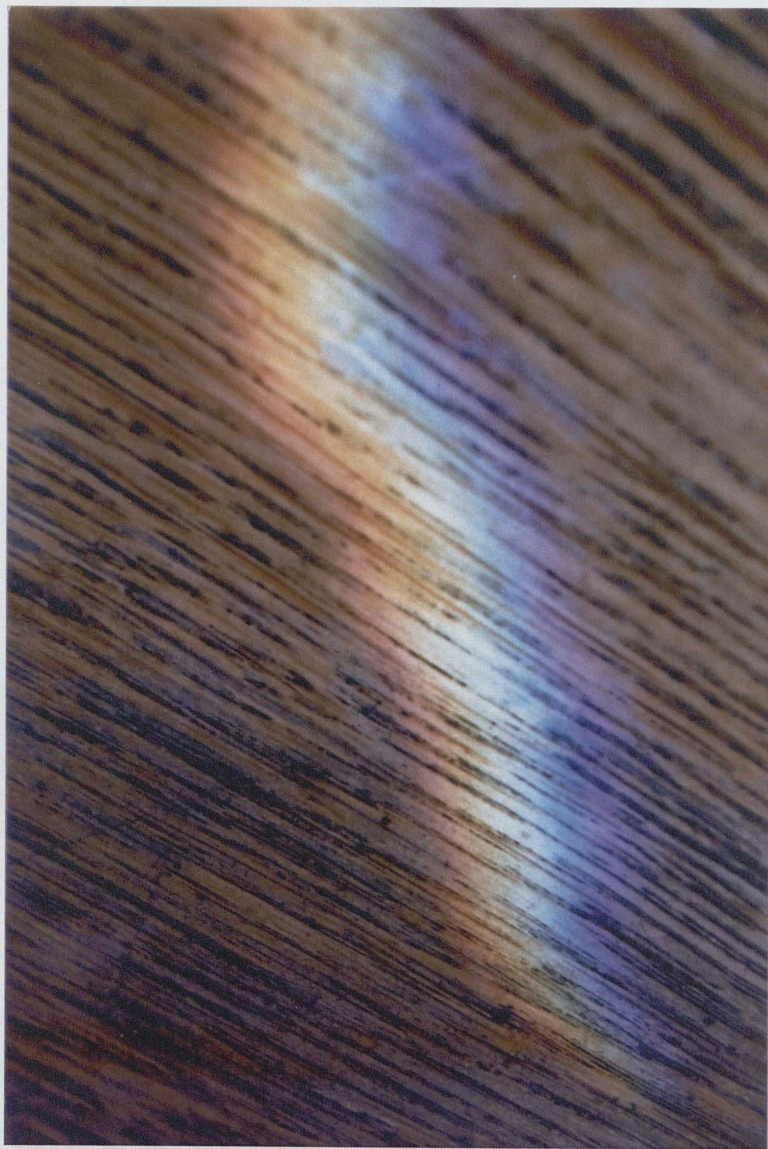
Tęcza [pryzmat]
