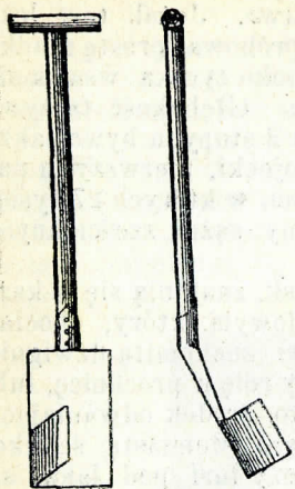
Szpadle do ręcznego rżnięcia torfu.
