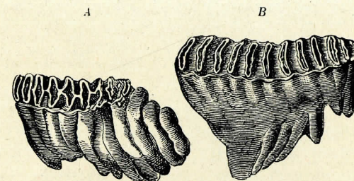
Ryc. 43. Ząb trzonowy. A — słonia afrykańskiego, B — indyjskiego.
