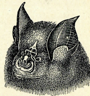
Ryc. 14. Głowa podkowca ( Rhinolophus ferrum-equinum ).
