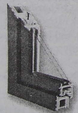
Przekrój trójkomorowy okna AWANS
