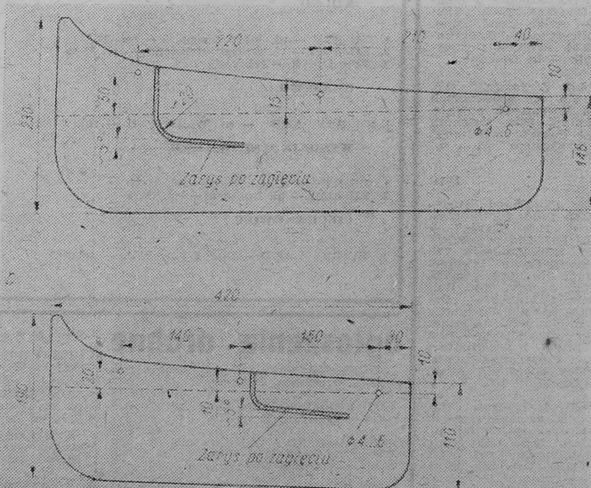
Rys. 224 Szkice wykonawcze przednich spojlerów a — samochodu PF 125p, b — samochodu PF 126p
