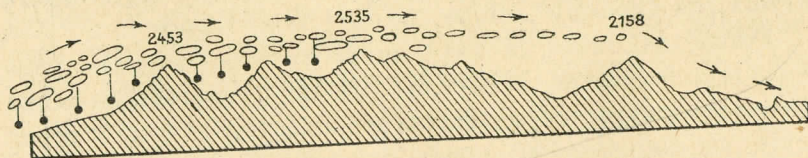
Ryc. 52. Wiatr halny w Tatrach. Gdy na południowych stokach Tatr powietrze podnosi się wgórę, para wodna w nim zawarta skrapla się. Pada tam deszcz. Tymczasem na stokach północnych powietrze, zstępując z grzbietów Tatr ku kotlinie Podhala, ogrzewa się, a para wodna w nim zawarta nie skrapla się, lecz ulatuje w powietrze. Wieją tu więc wiatry suche i ciepłe, które powodują na wiosnę szybkie tającie śniegu w górach i gwałtowne wzbieranie potoków.
