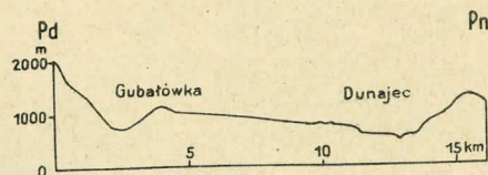
Ryc. 58. Przekrój przez Podhale. Widać, jak kraj obniża się zwolna ku północy.
