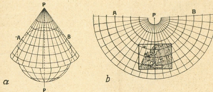
Ryc. 2. a — stożek nałożony na kulę; b — pobocznica stożka rozplaszczona i układ południków i równoleżników w siatce stożkowej.
