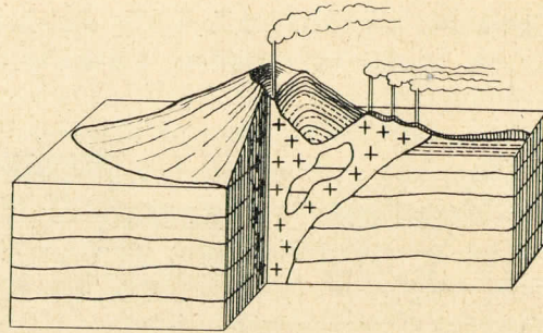
Ryc. 25. Przekrój wulkanu.
