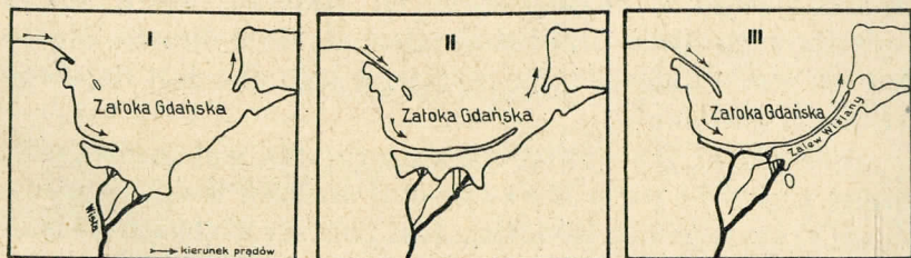
Ryc. 178. Schemat powstania mierzei.
