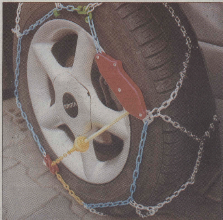
Łańcuchy o drobnych ogniwkach (10 mm) mają dużą wytrzymałość. Mechanizm z boku koła samoczynnie likwiduje luz.
