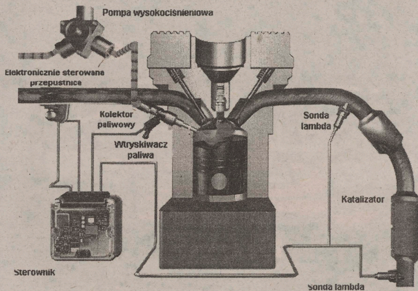
System bezpośredniego wtrysku benzyny Bosch Motronic MED 7
