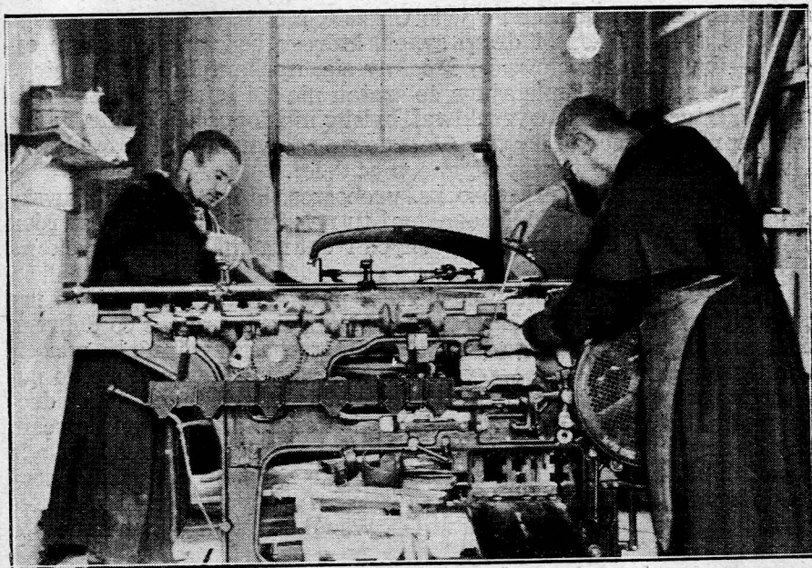
Bracia w Mugenzai no Sono montują falcówkę (maszynę do składania arkuszy „Rycerza“).
