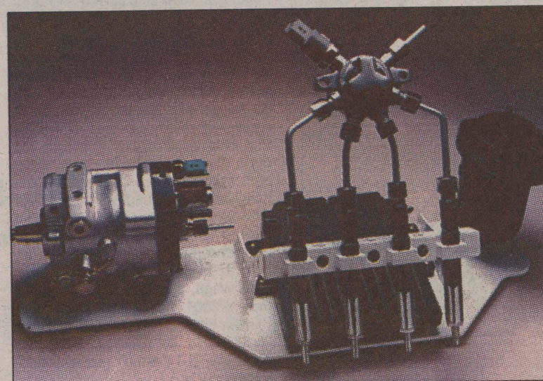
Układ zasilania opracowany wspólnie z firmą Delphi
