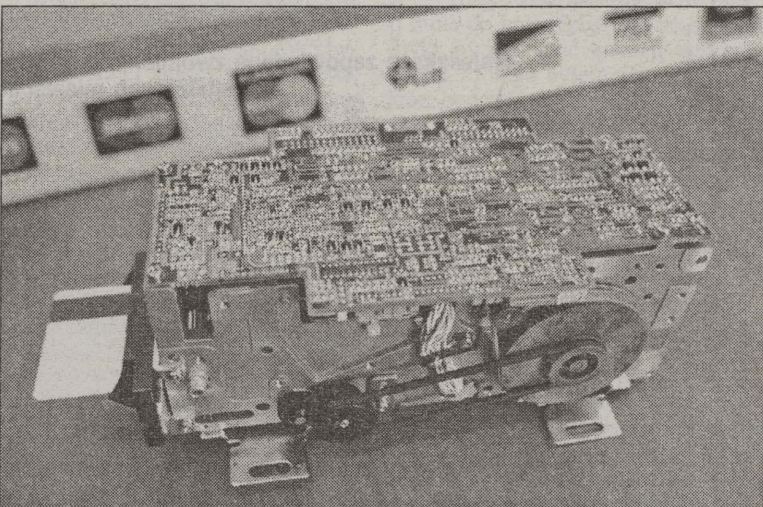
Przy pomocy tego urządzenia elektronicznego złodzieje kopiowali skradzione zapisy na tzw. białych plastikach
