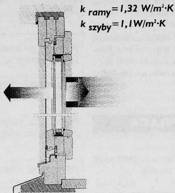
Współczynnik przenikania ciepła w oknach 2-szybowych, jednoramowych SKJ-94
