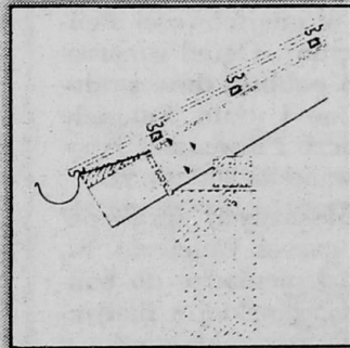
Okap
