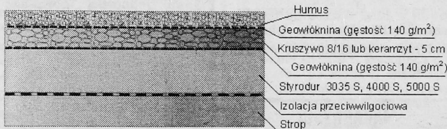
Dach zielony jako dach odwrócony
