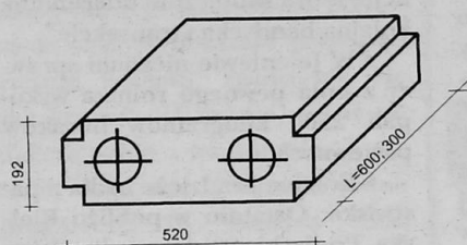
Pustak stropowy SKB
