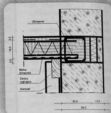
Oparcie belki na ścianie zewnętrznej
