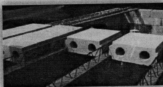
Układanie pustaków na belkach stropowych
