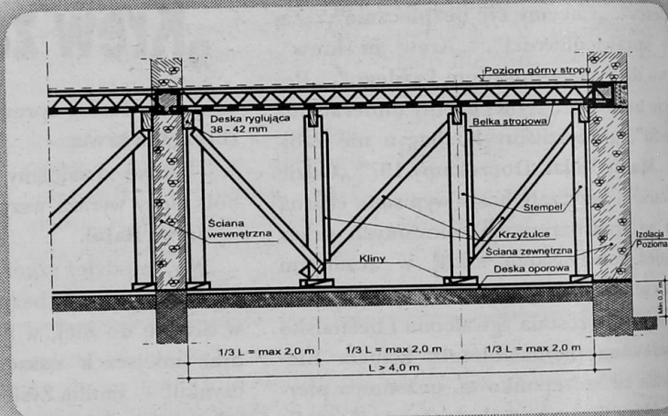
Układanie pustaków na belkach stropowych
