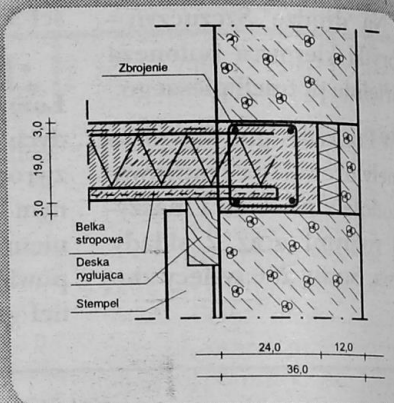
Oparcie belki na ścianie zewnętrznej
