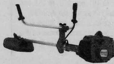
husqvarna 343R 45.0 cm 3 - 2.0 kW / 2.7 KM - 8.2 kg
