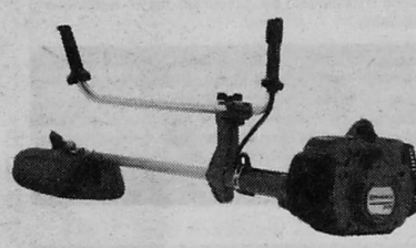
husqvarna 343R 45.0 cm 3 - 2.0 kW / 2.7 KM - 8.2 kg
