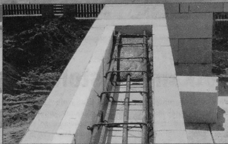
Prawidłowo wykonane i zazbrojone nadproże z elementem ocieplającym.
