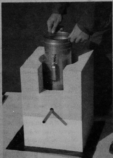
Montaż podstawy komina wraz z wyczystką i miską na kondensat.
