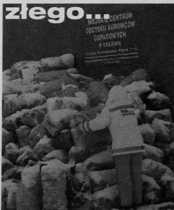
W Miejskim Centrum Odzysku Surowców Odpadowych przy ul. Ekologicznej śmieci z domowej selekcji grajewian są przygotowywane do recyklingu
