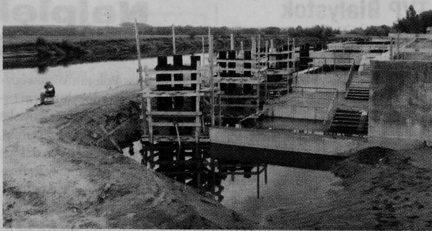
Po usunięciu ziemi między nabrzeżem a rzeką, rzeka będzie szersza w tym miejscu około 30 m
