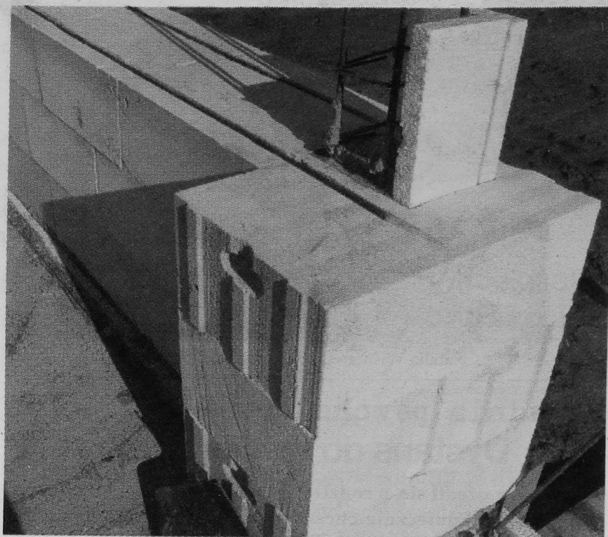
Ściana jednowarstwowa - beton komórkowy WP 42 x 24 x 59 (G430)
