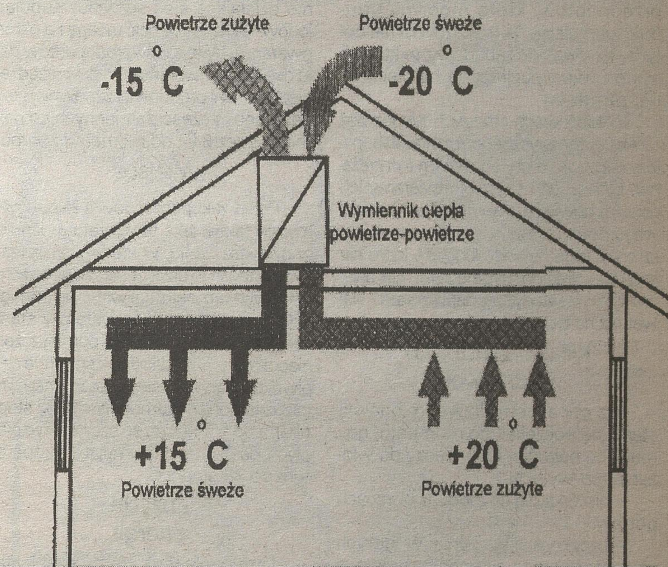
Urządzenia do odzysku ciepła z wentylacji montuje się z reguły w okolicach kalenicy lub pod skosami dachu (na zdjęciu) – tam gdzie z reguły jest niewykorzystana powierzchnia budynku
