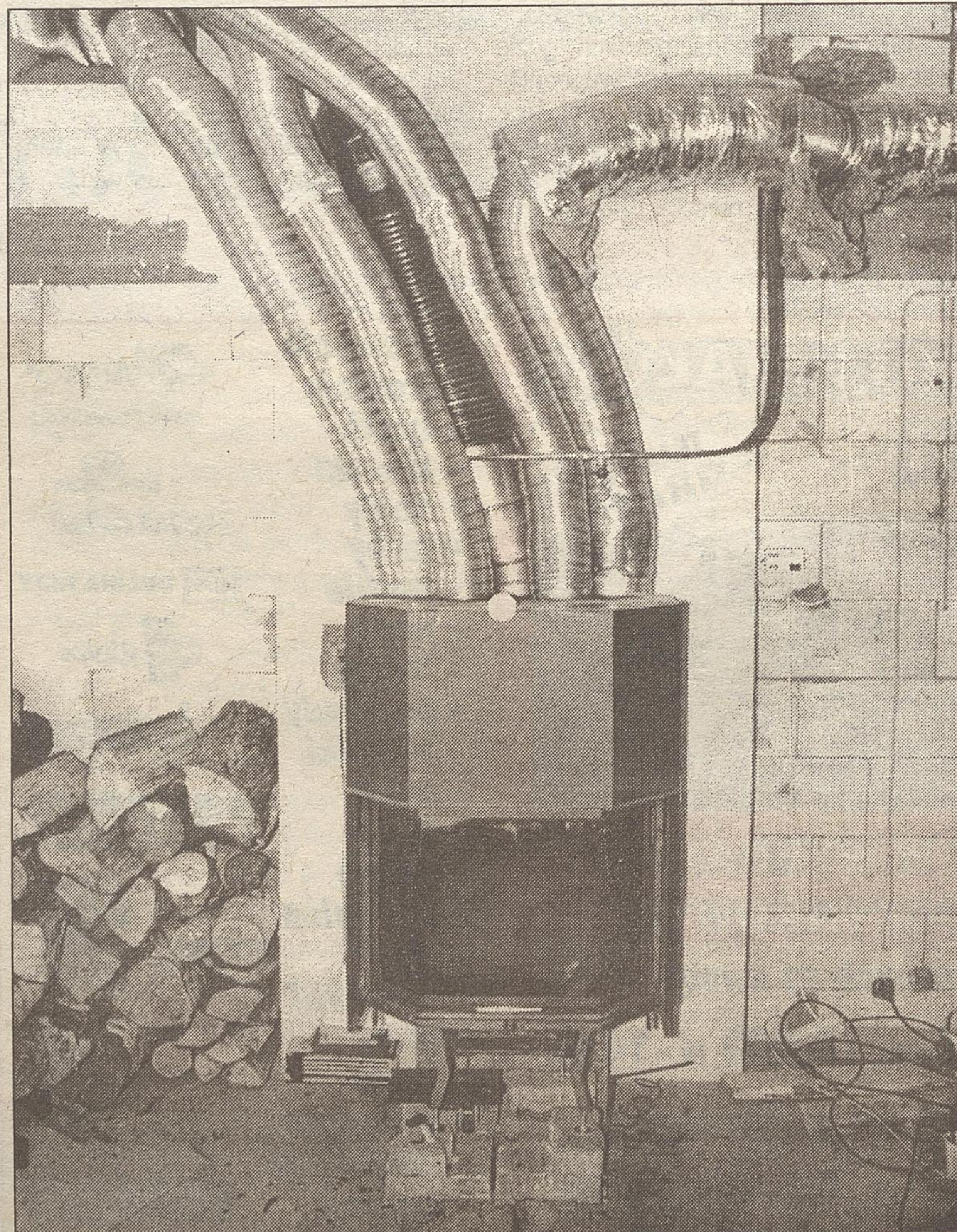
Tak wygląda niezabudowany jeszcze kominiek podłączony do systemu wentylacji z odzyskiem ciepła, dzięki temu ciepło z niego jest rozprowadzane po całym budynku
