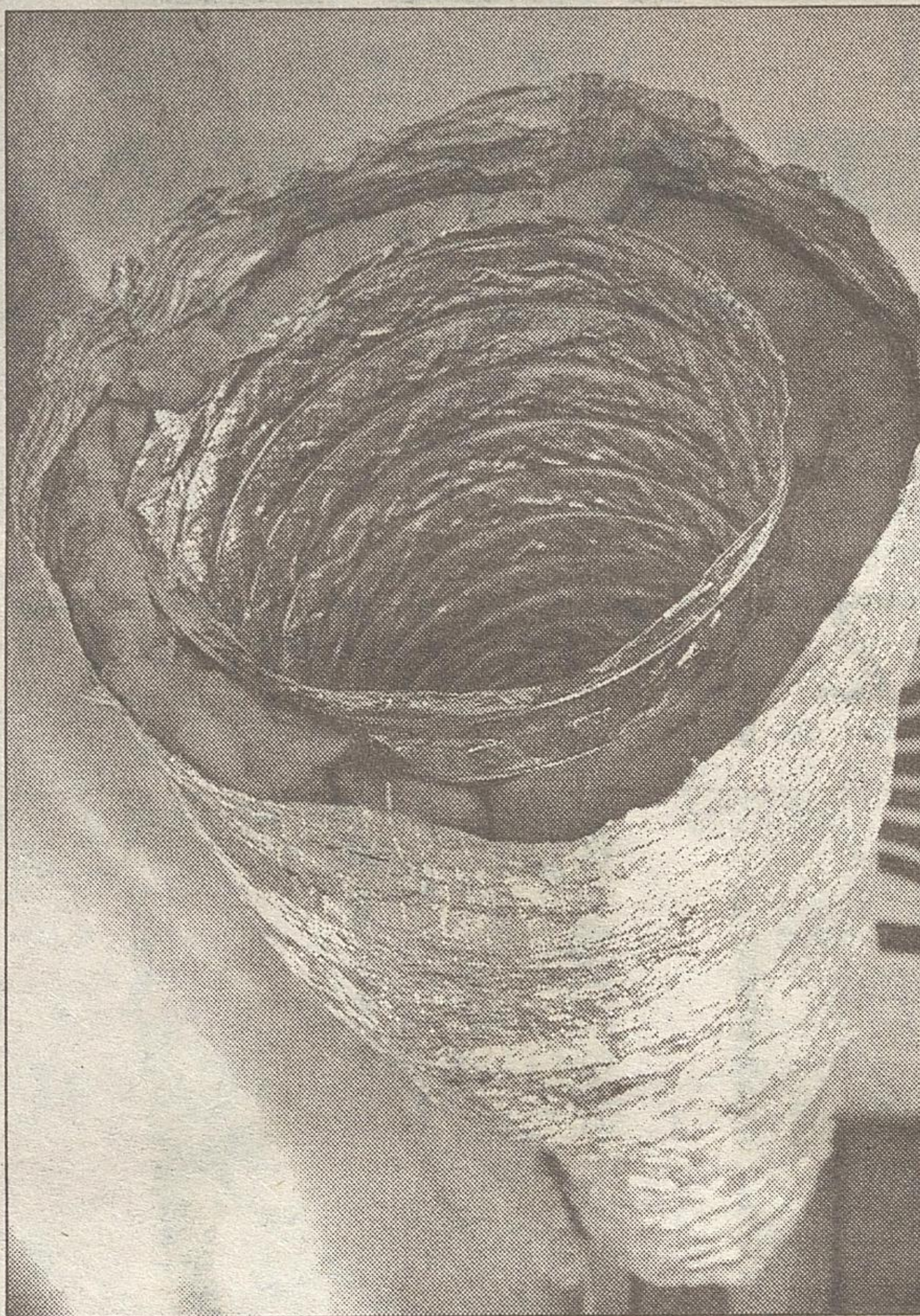
Rura zaizolowana (z lewej) i niezaizolowana – druga odprowadza ciepłe powietrze, pierwsza – doprowadza zimne powietrze do wymiennika
