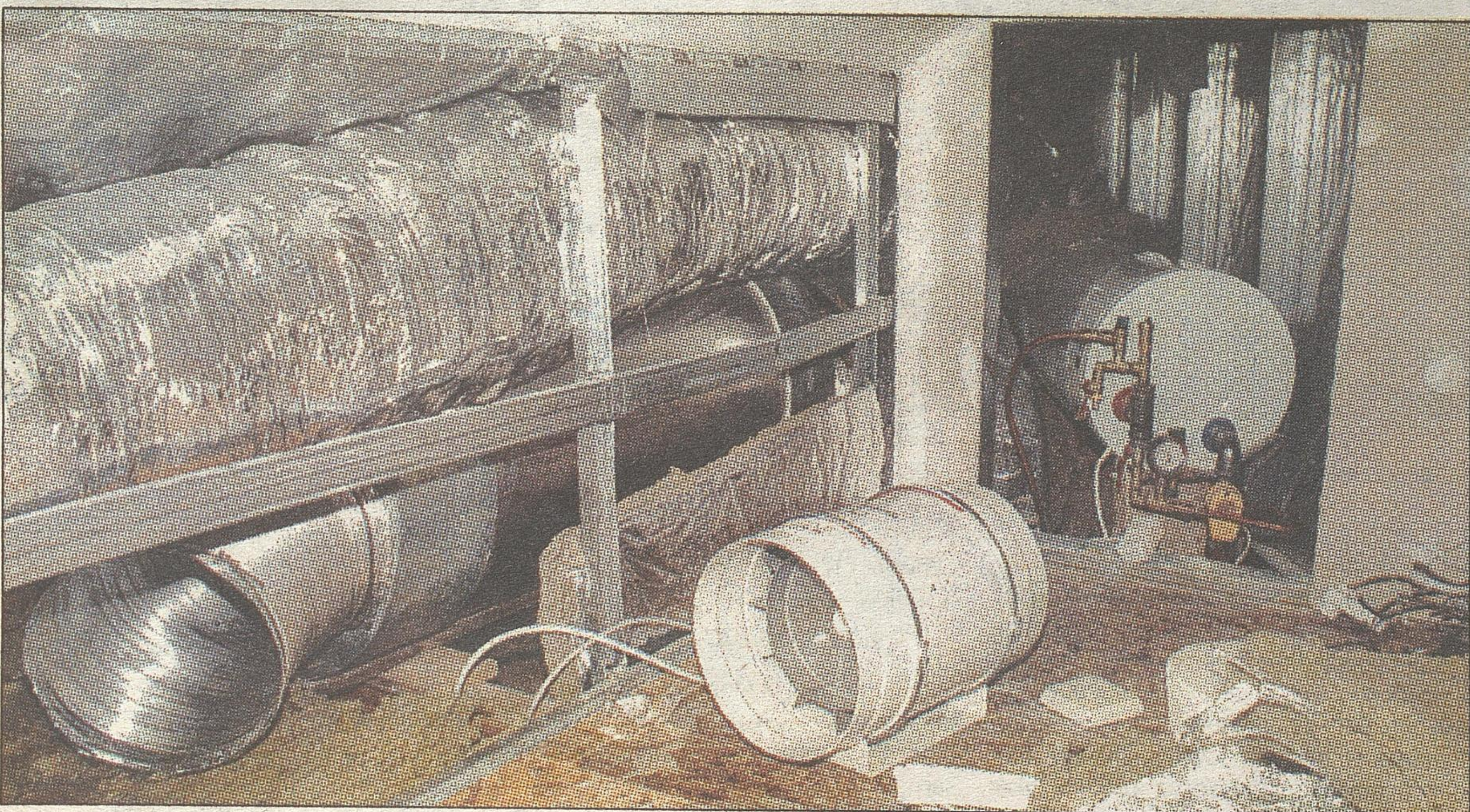
Urządzenia do odzysku ciepła z wentylacji montuje się z reguły w okolicach kalenicy lub pod skosami dachu (na zdjęciu) – tam gdzie z reguły jest niewykorzystana powierzchnia budynku
