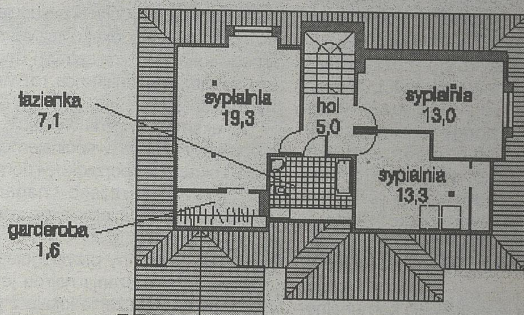
rzut poddasza
