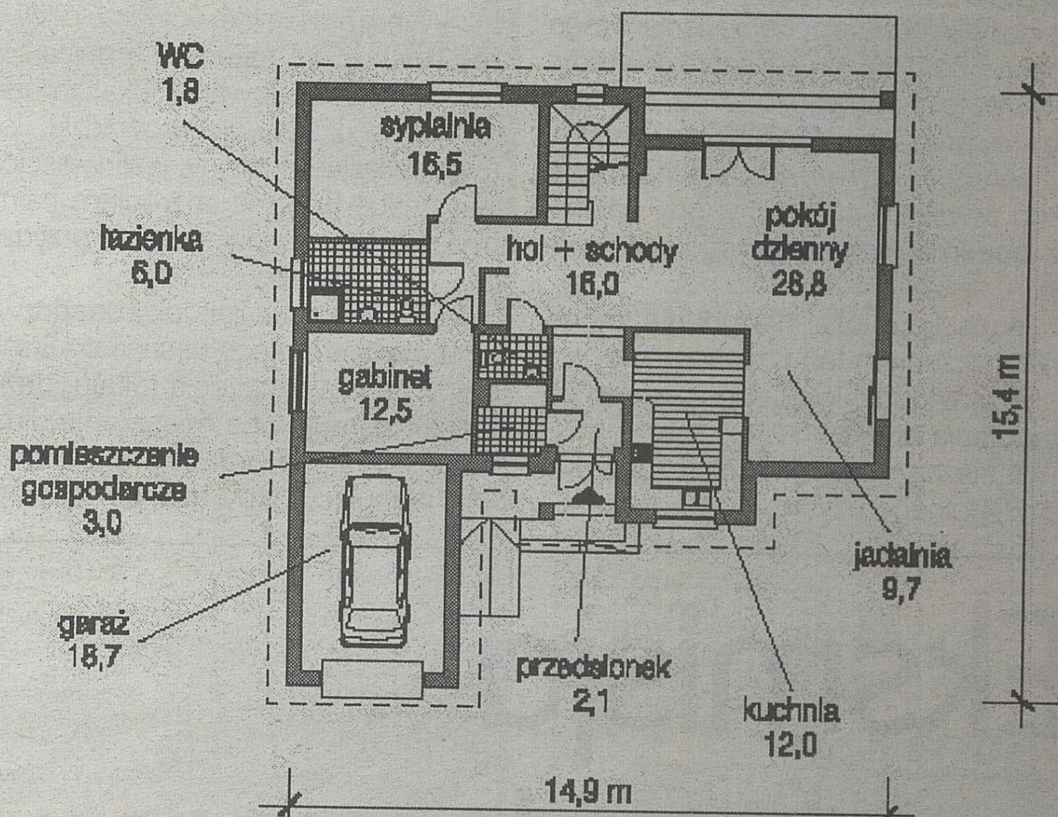
rzut parteru
