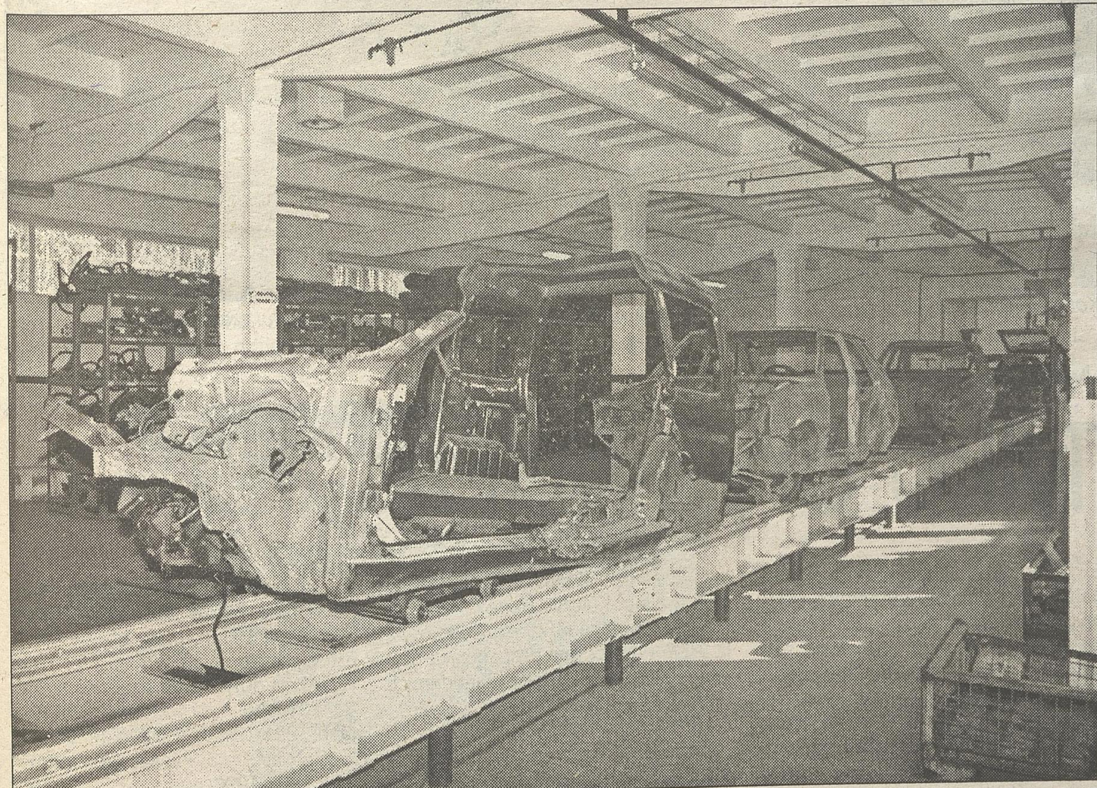
Taśma demontażu nadwozi przeznaczonych do złomowania
