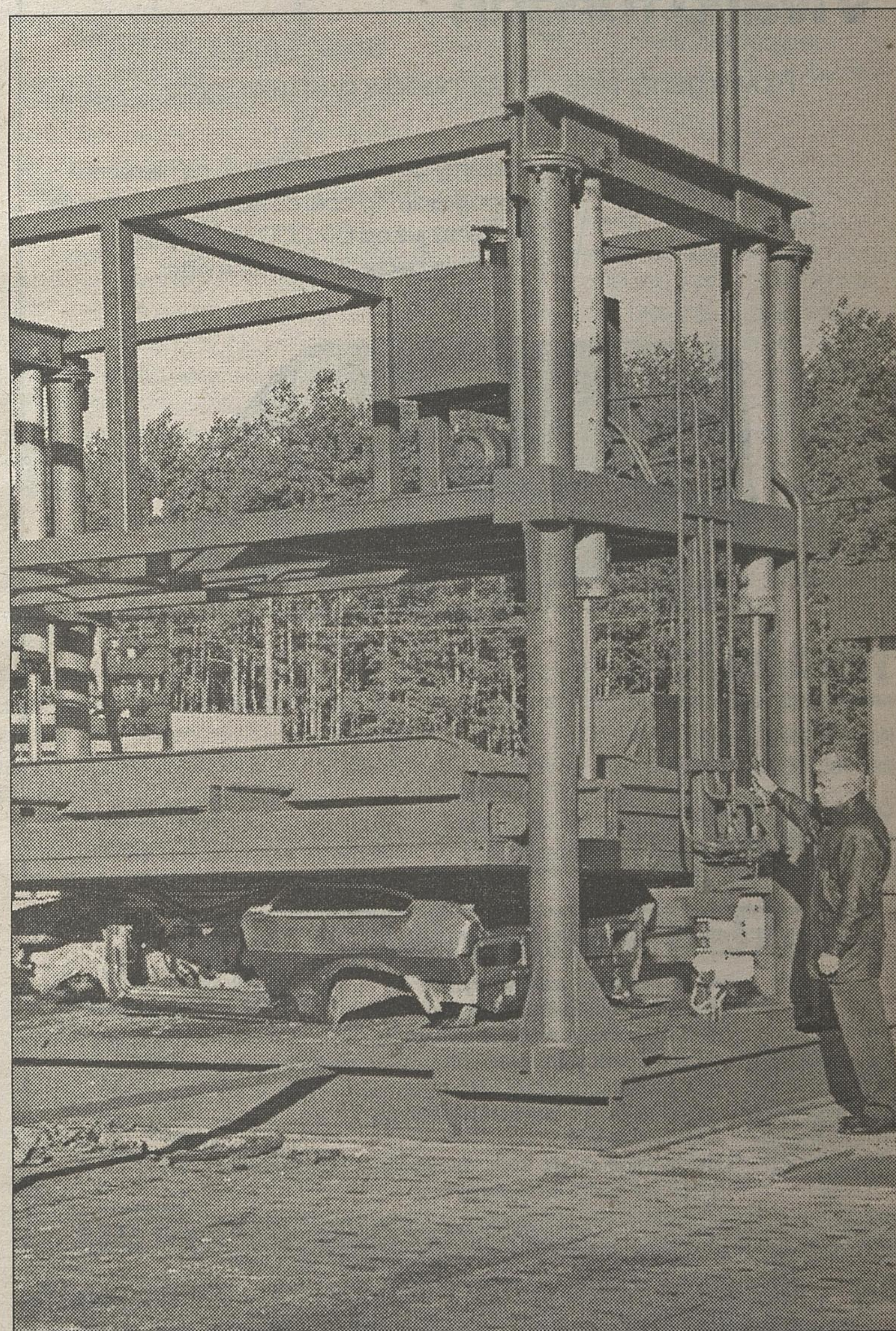
Prasa do zginiatania nadwozi przed wysyłką do huty
