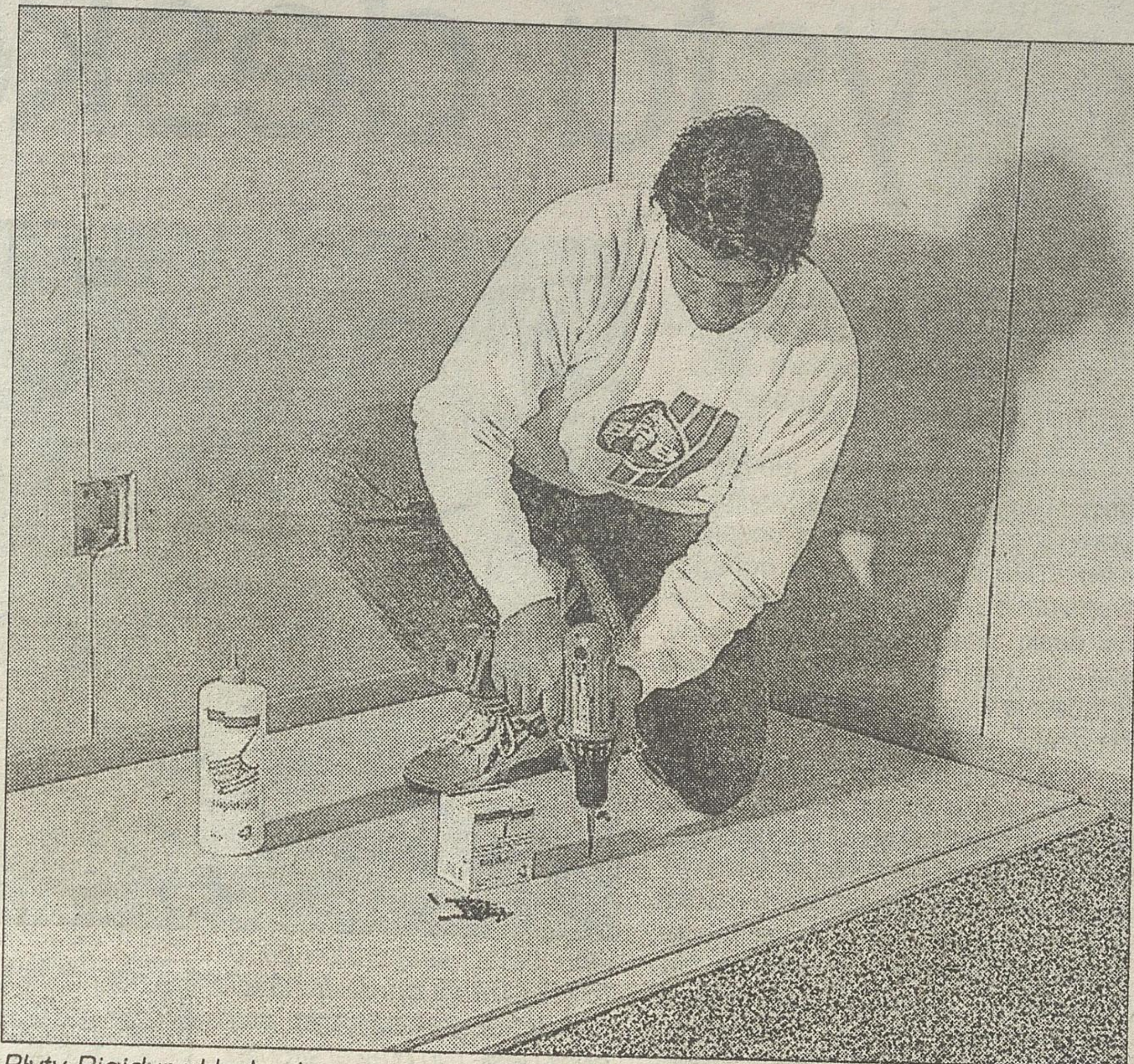
Płyty Rigidur układa się zaczynając od lewej strony ściany przeciwległej do drzwi
