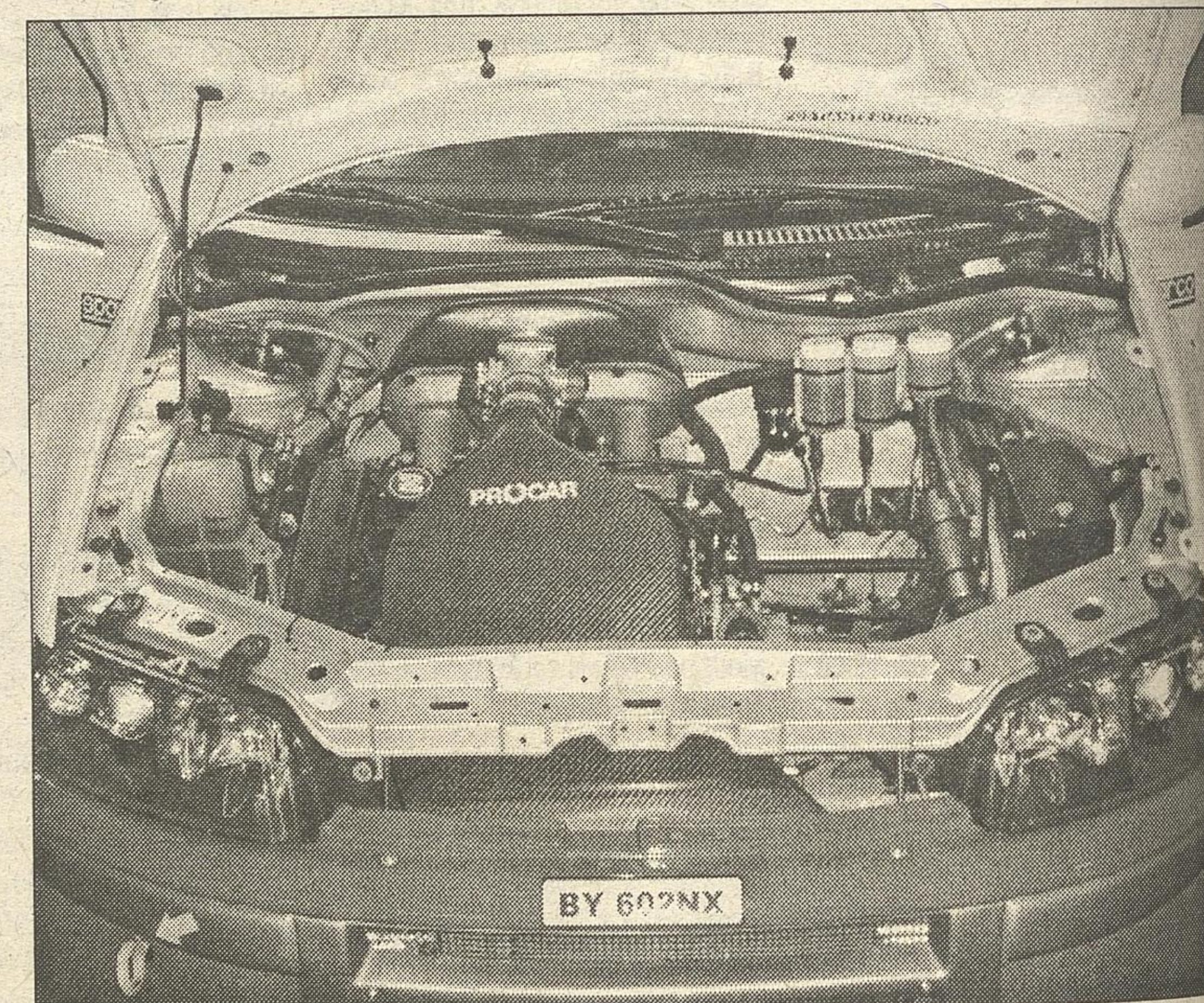
Komora silnika, wyraźnie widać nową konstrukcję układu doprowadzenia powietrza
