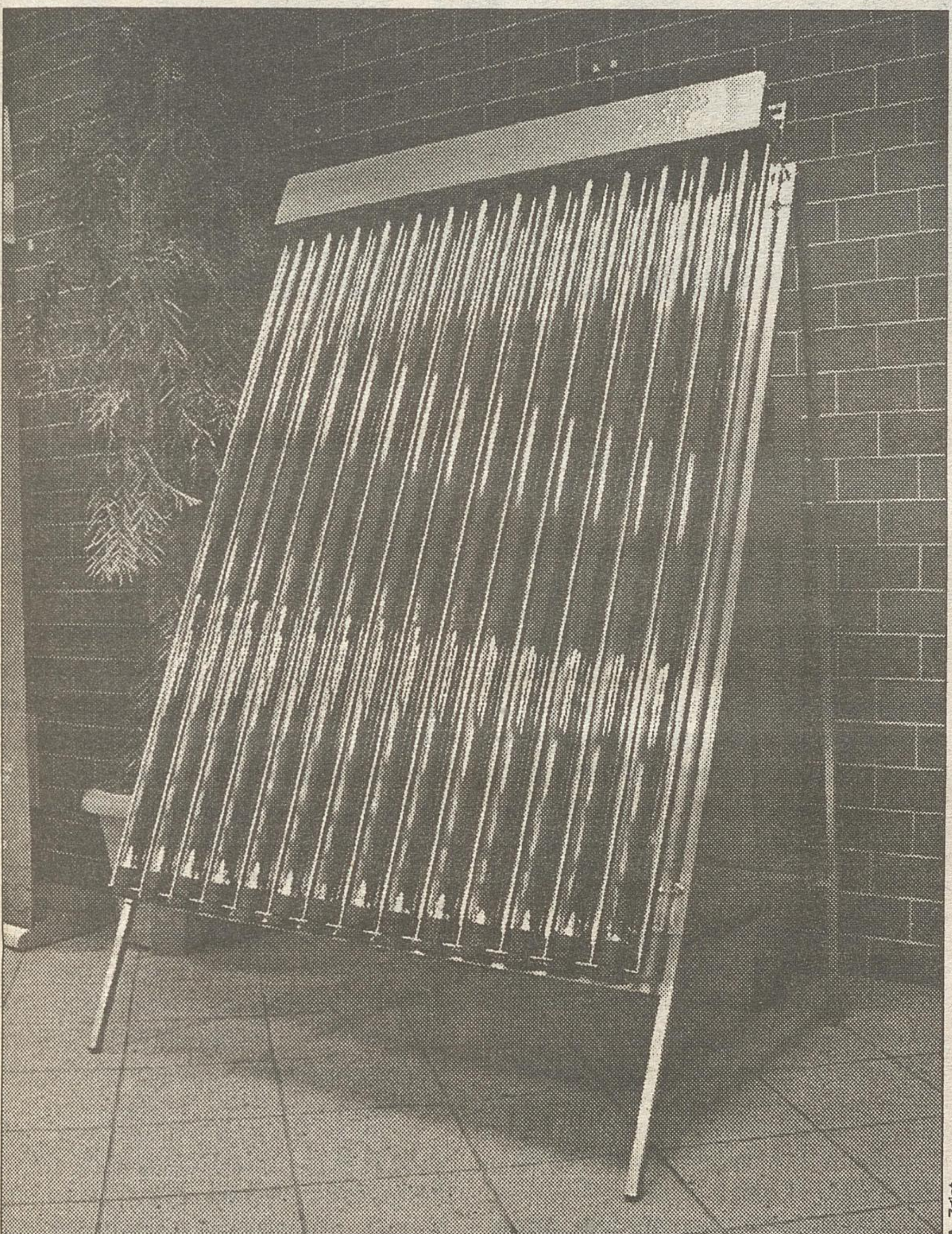
Słoneczne kolektory próżniowe składają się nie tylko z kolektora (na zdjęciu), ale także całej towarzyszącej automatyki
