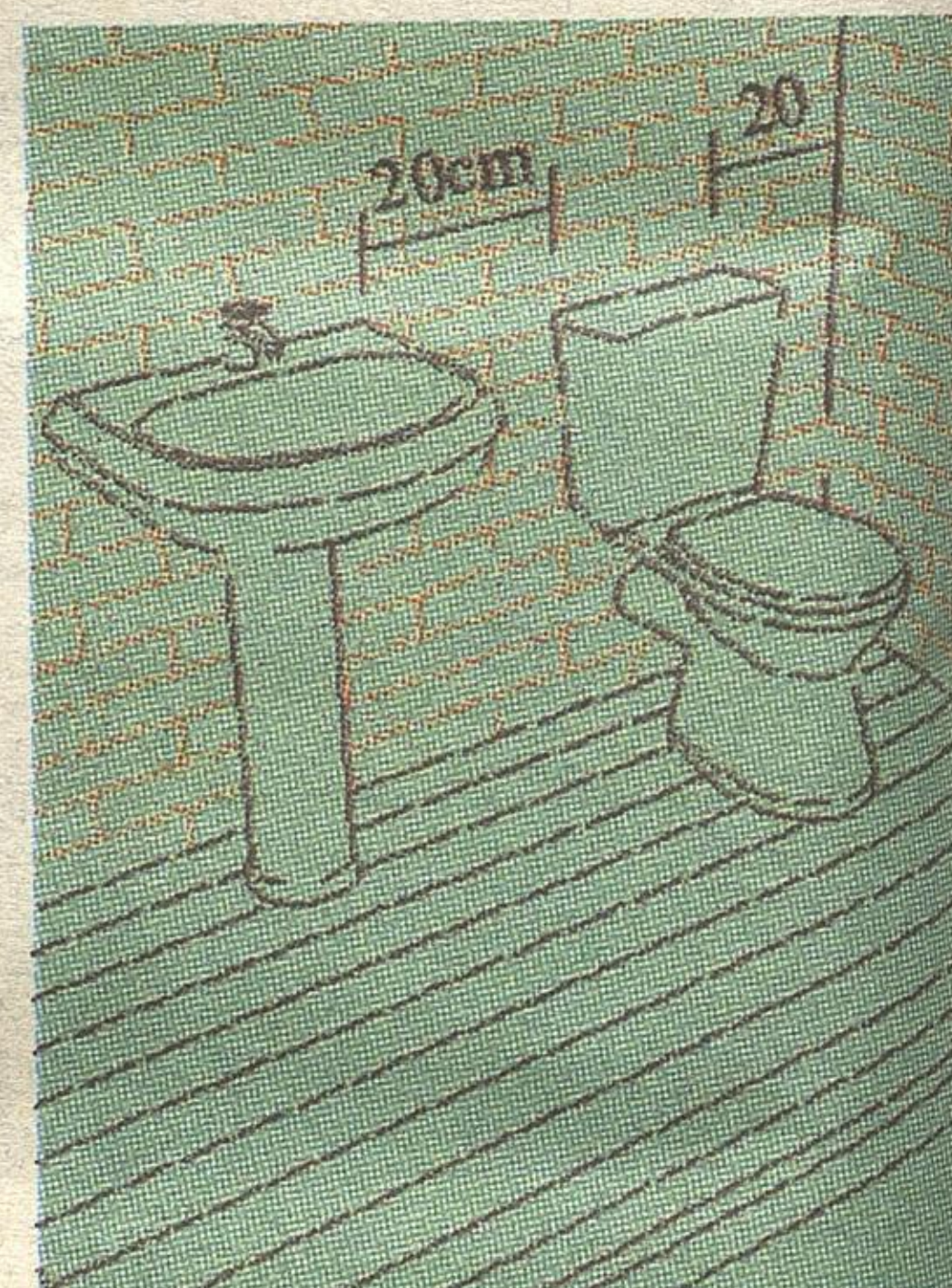
Minimalne odległości między elementami toalety
