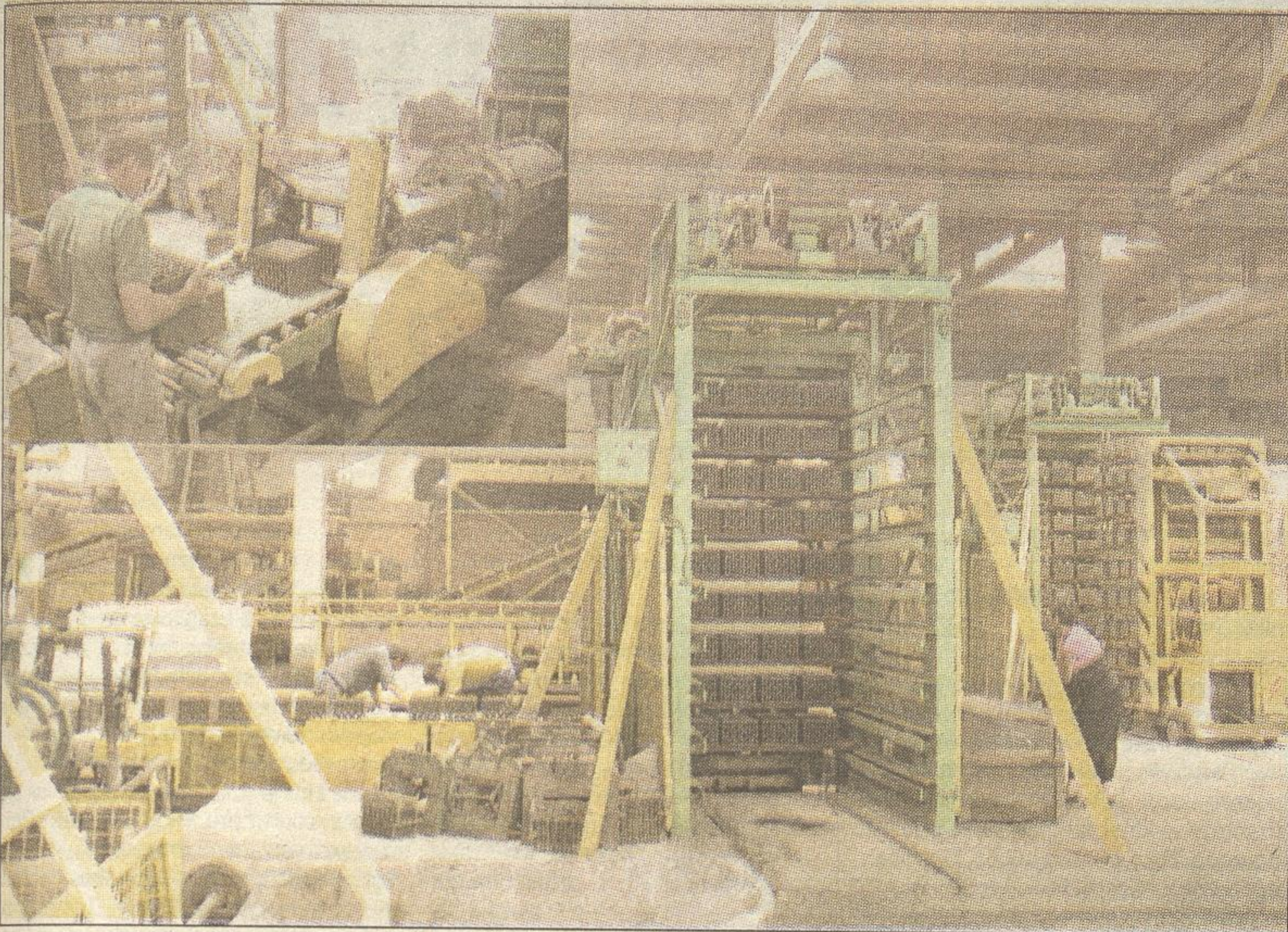
Jakość ceramiki po wyjściu spod prasy jest kontrolowana, cegły są przygotowywane do suszenia
