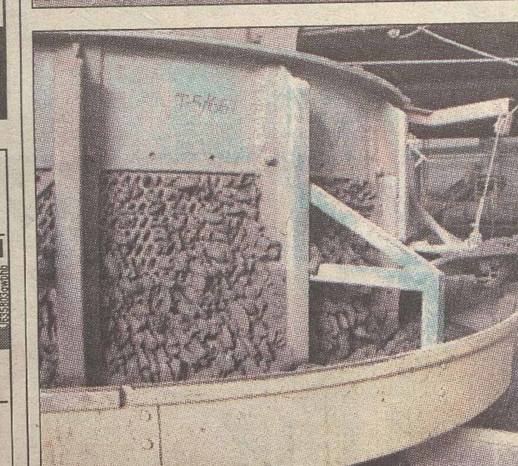
Glina zmieszana z dodatkami piasku i pyłu ceglanego składowana jest przez dwa tygodnie w tzw. dołowniku, skąd trafia do tzw. przeciaraka
