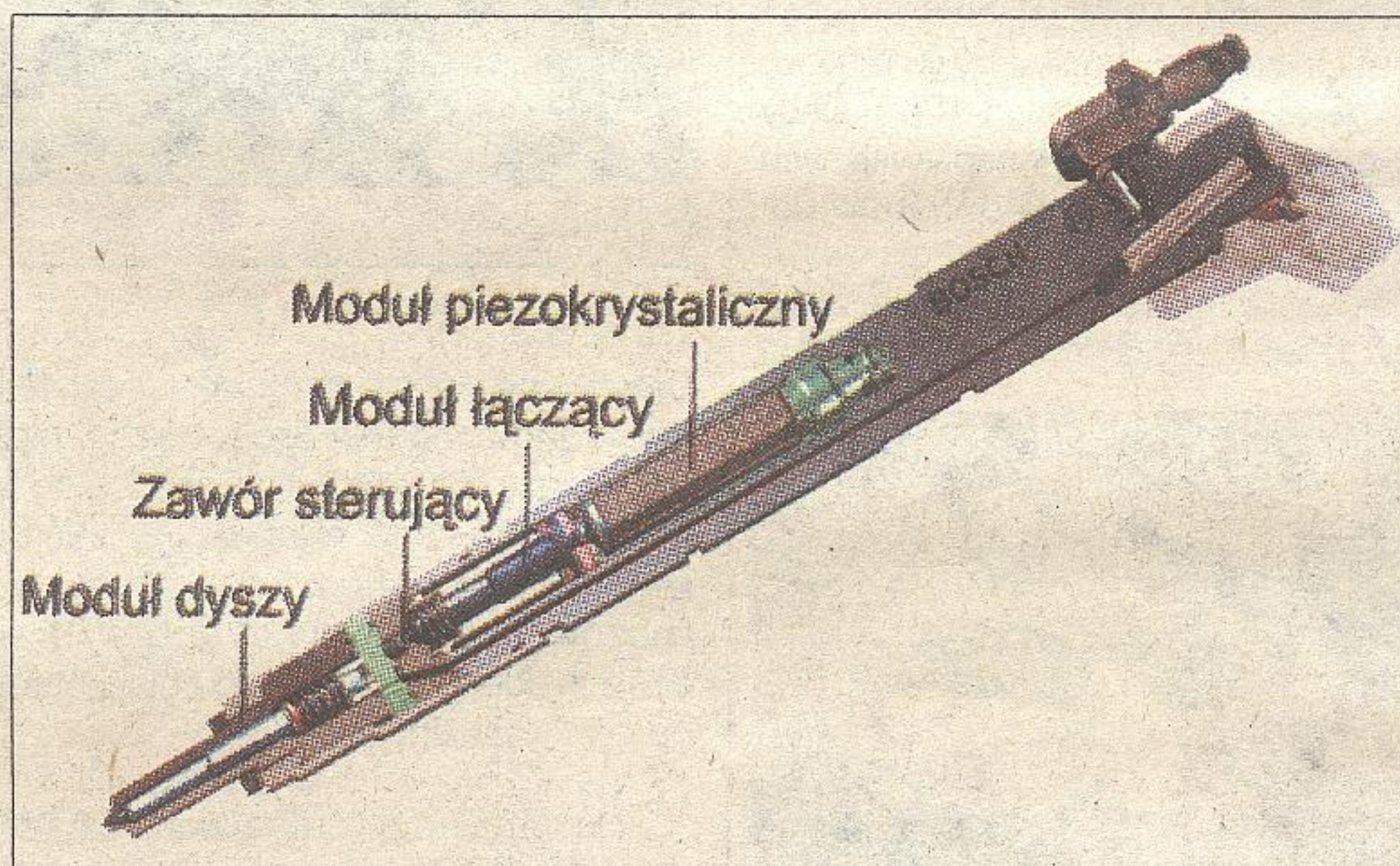
Wtryskiwacz piezokrystaliczny (Inline Injector)
