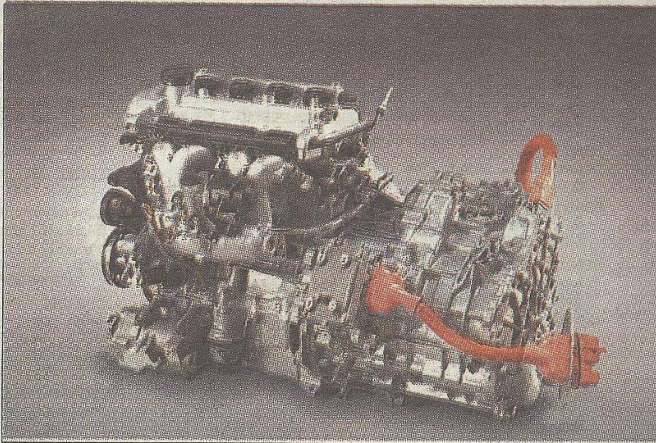
Zespół napędowy Priusa THS
