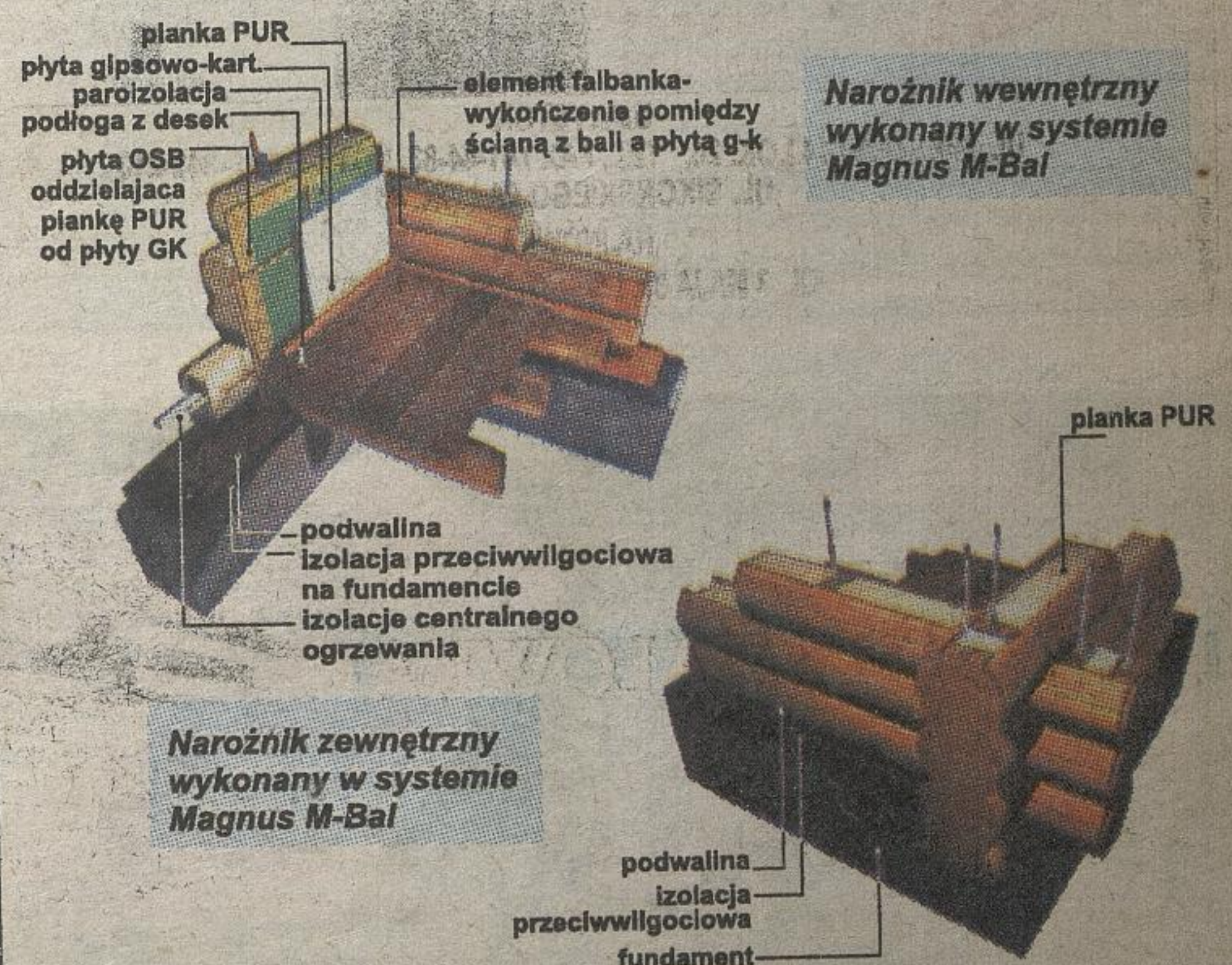
Przekrój przez ścianę wykonaną w systemie M-Bal pokazujący dwa warianty wykończenia ściany od wewnątrz: ścianę zarówno z zewnątrz jak i wewnątrz wykonaną z bala prefabrykowanego, oraz ścianę przystosowaną od wewnątrz do wykończenia wnętrza płytą gipsowo-kartonową
