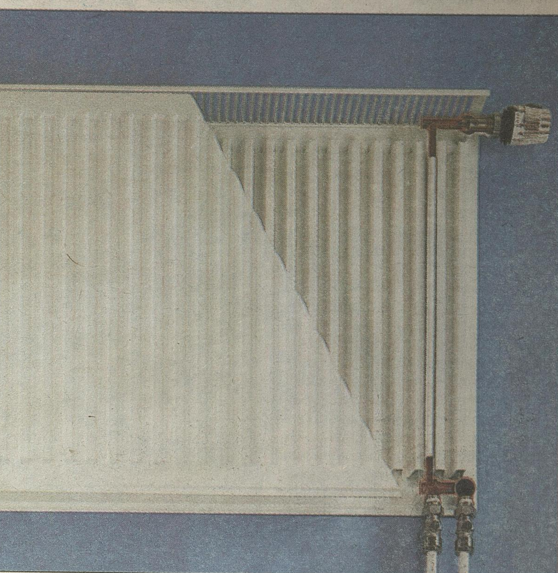
Przekrój grzejnika płytowego
