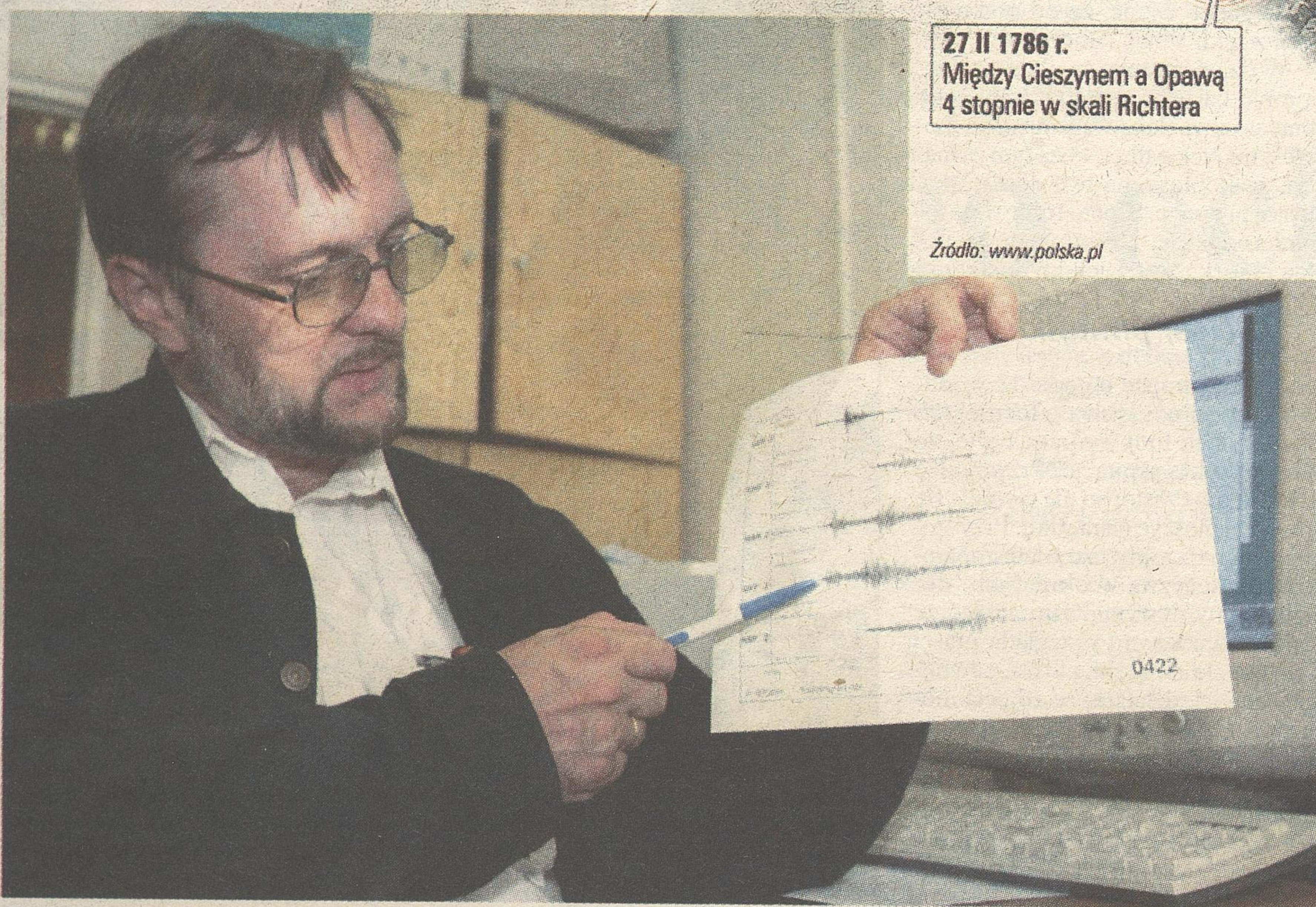
Dr Paweł Wiejacz demonstruje wykres wstrząsów seismicznych, jakie miały miejsce w Polsce
