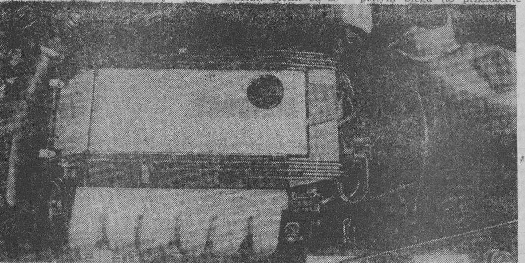
„Serce” Passata — sześciocylindrowy widlasto-rzędowy silnik o mocy 174 KM.
