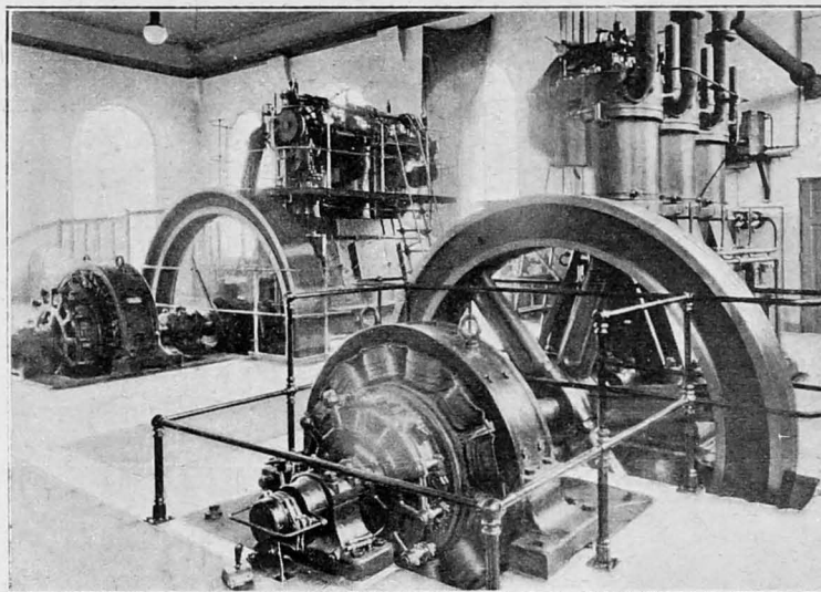
Motory Diesla w dużej sali.
