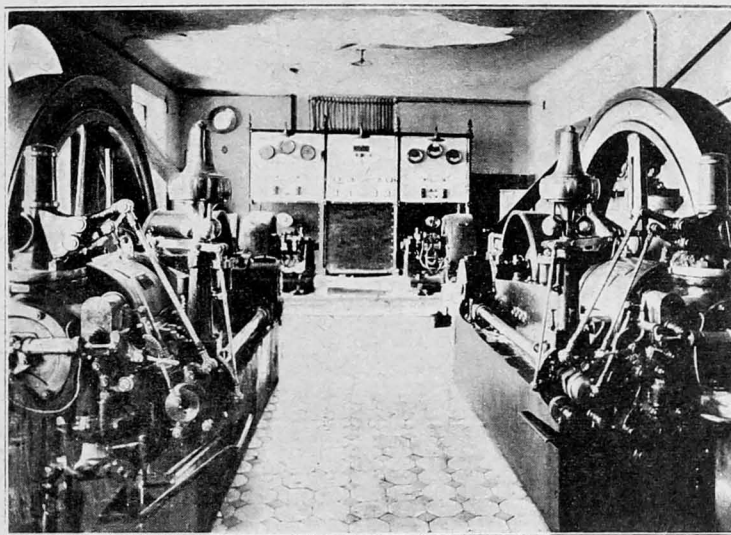
Pierwsze mniejsze motory na gaz ssany (35 koni).
