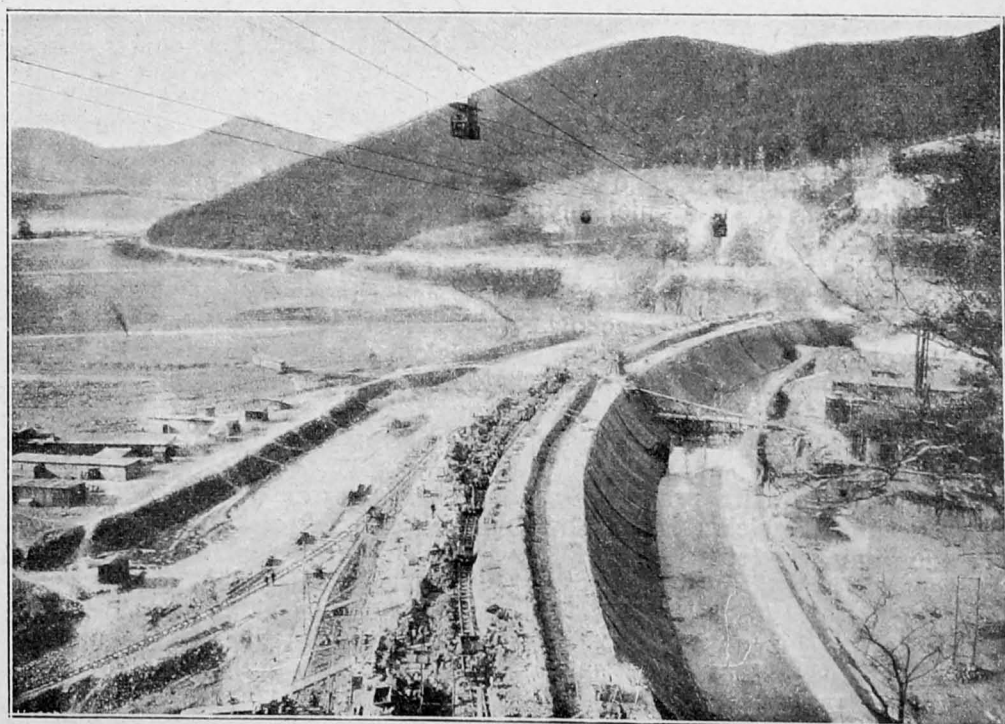
Budowa ściany sztucznego jeziora.
