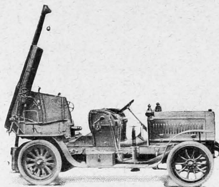
Francuskie działo przeciwbalonowe, pomysłu kapitana Houberdona.
