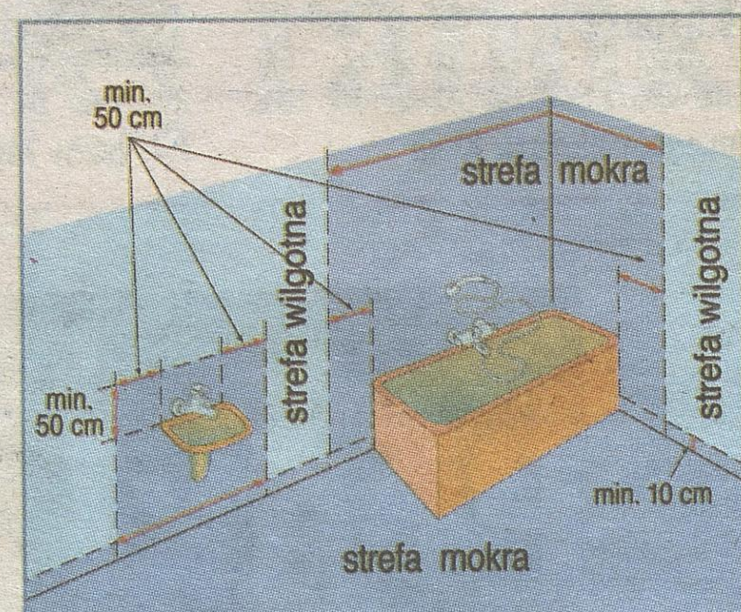
Rozmieszczenie stref mokrych i wilgotnych wokół wanny i umywalki
