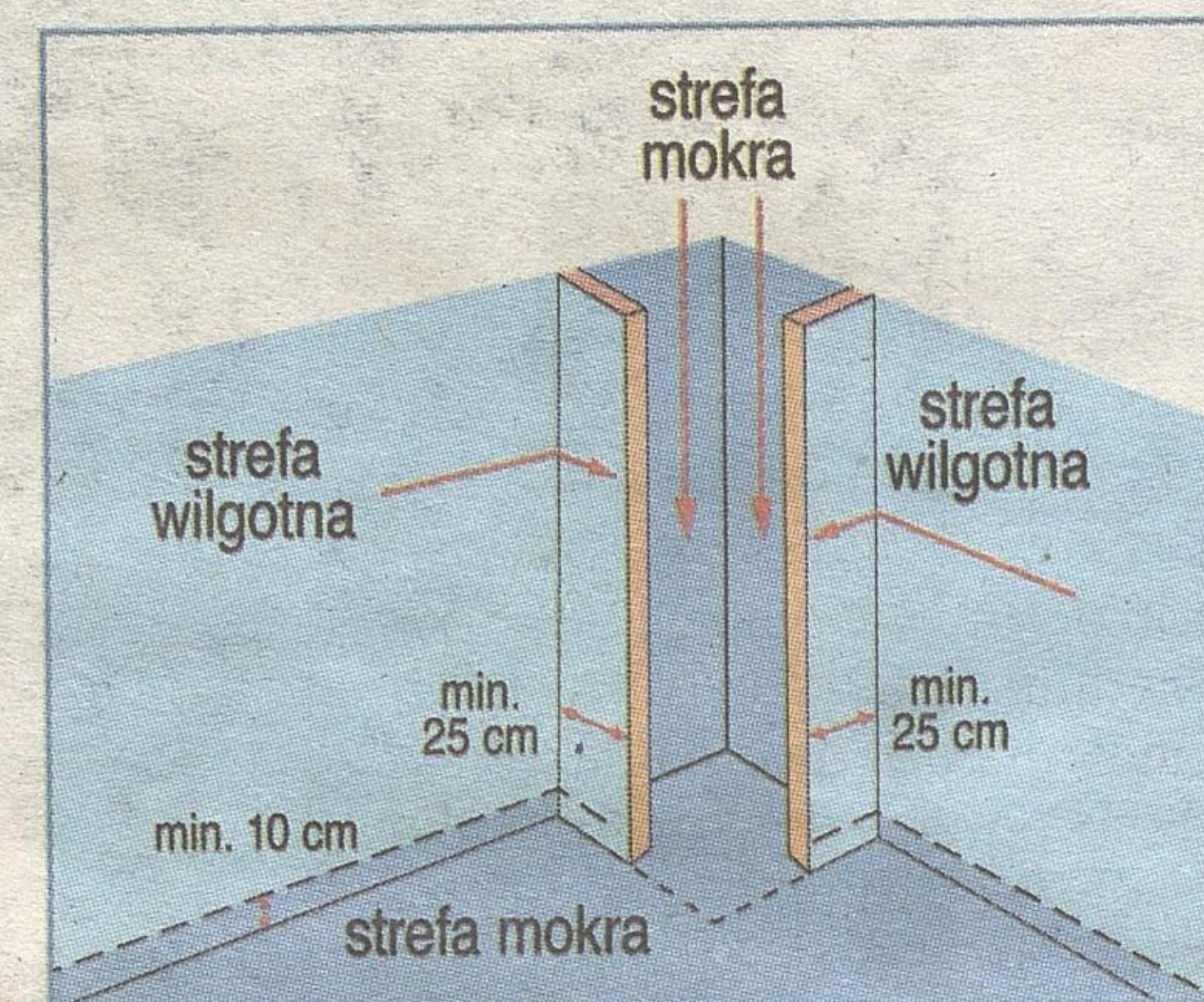
Rozmieszczenie stref mokrych i wilgotnych wokół kabiny prysznicowej
