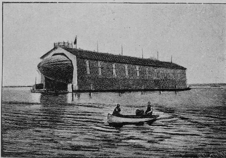
Przystań balonu Zeppelina na jeziorze Badeńskim.
