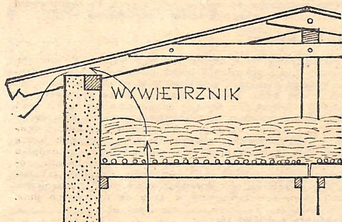
Górna część kurnika z wbudowanym stropem ażurowym. Strzałki pokazują jak zużyte, wilgotne powietrze przedosta- je się przez słomę i uchodzi na zewnątrz.
