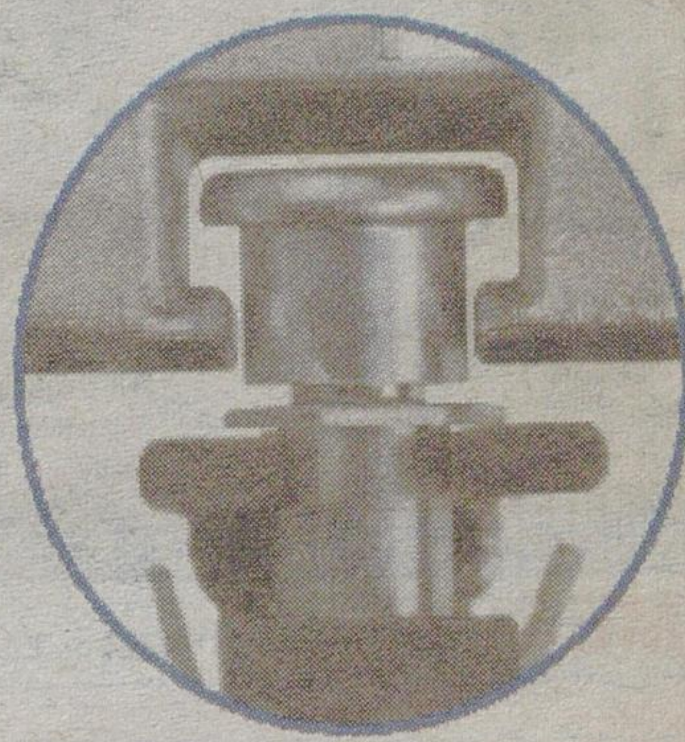
Czop i.S. wraz z zaczepem antywyważeniowym Safety Plus
