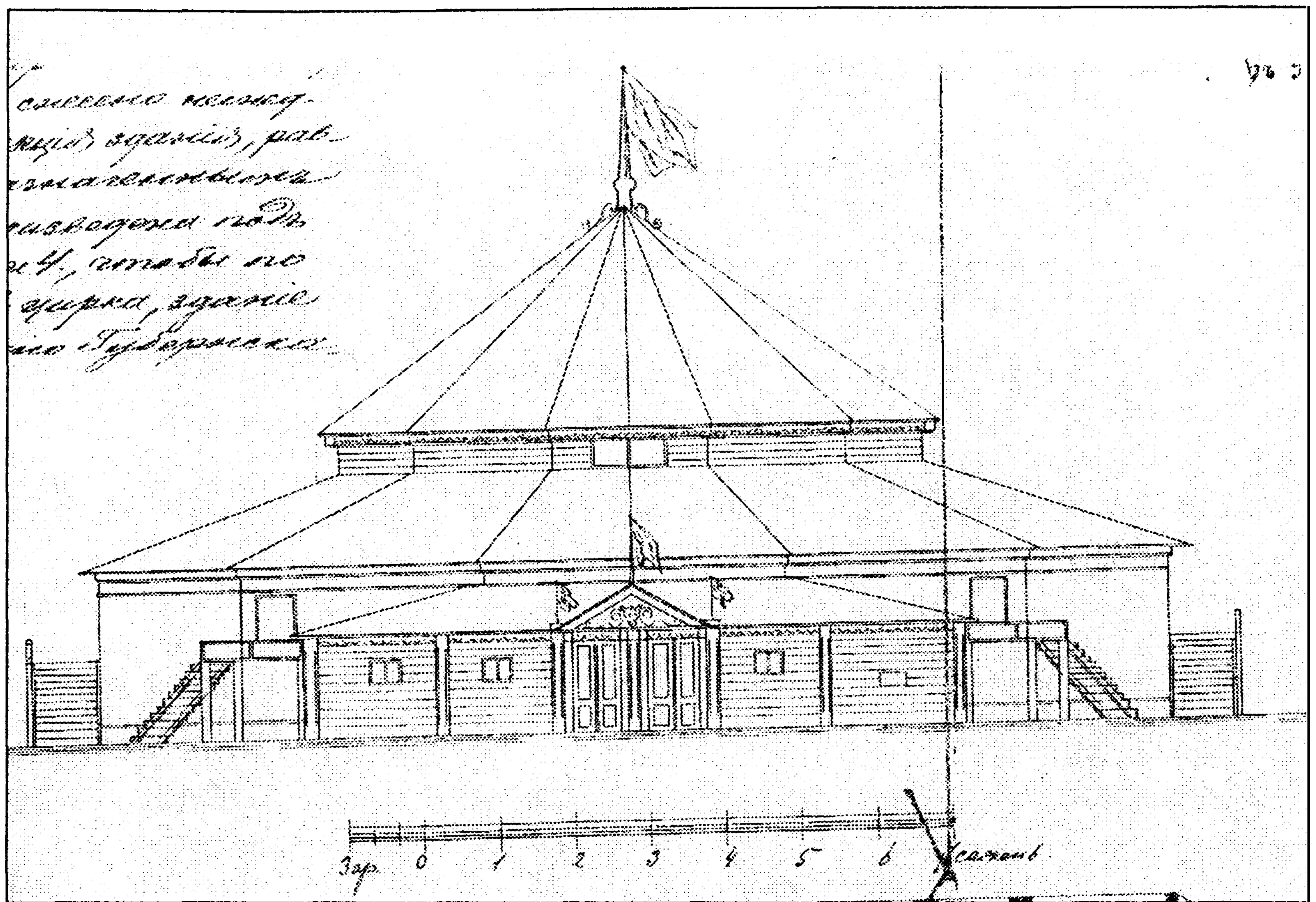
il.5. Projekt drewnianego cyrku Iwana Knaupa w Białymstoku, arch, Płotnikow, 1894
