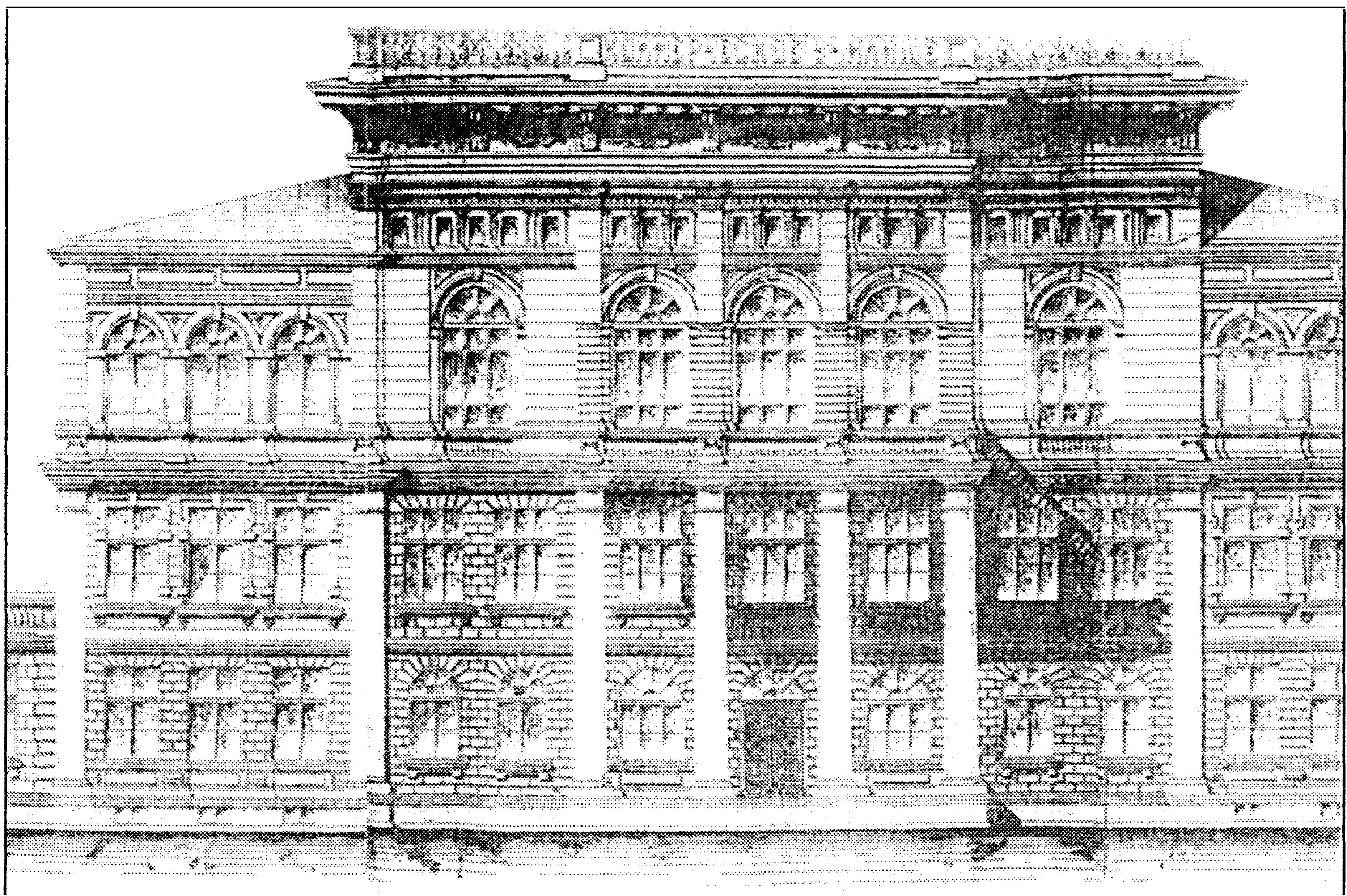
il.2. Projekt przebudowy domu Moesa przy ul. Warszawskiej na szkołę handlową, arch. Bieriezin, 1903.
